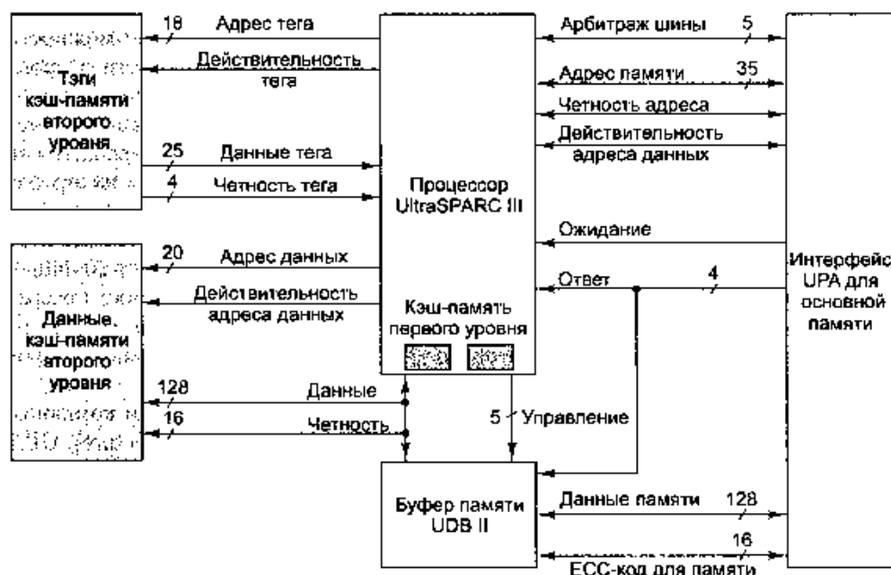
Рис. 3.45. Базовая структура системы UltraSPARC III
