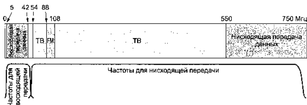
Рис. 2.36. Распределение частот в стандартной системе кабельного телевидения с возможностью доступа в Интернет
