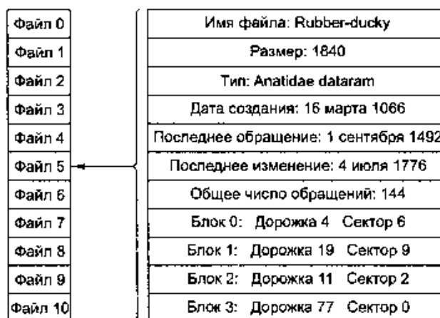
Рис. 6.20. Пользовательский каталог и структура одного из типичных файлов
