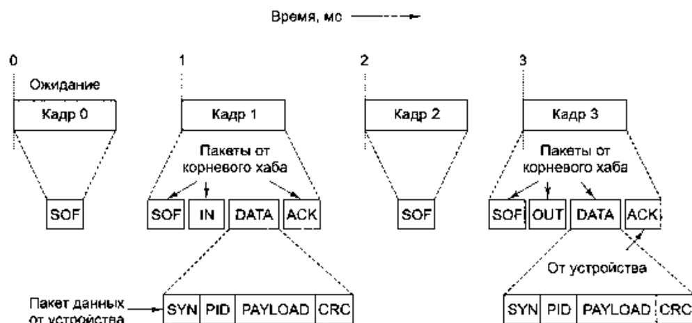
Рис. 3.55. Корневой хаб шины USB передает кадры каждую миллисекунду
