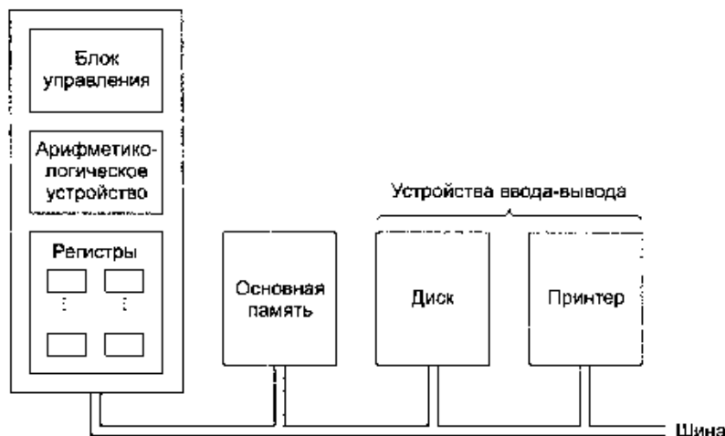
Рис. 2.1. Схема компьютера с одним центральным процессором и двумя устройствами ввода-вывода
