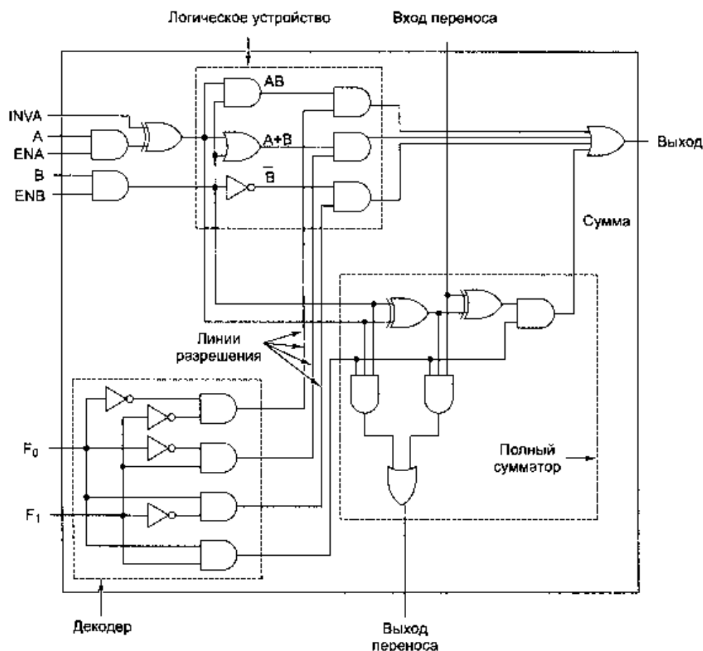
Рис. 3.18. Одноразрядное АЛУ
