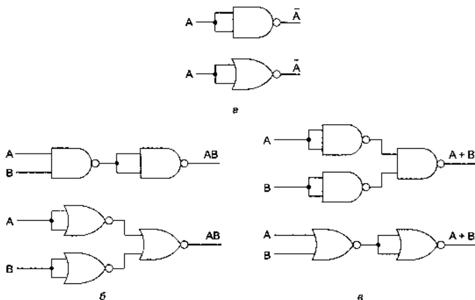
Рис. 3.4. Конструирование вентилях НЕ (а), И (б) и ИЛИ (в) только на базе вентилля НЕ-И или НЕ-ИЛИ
