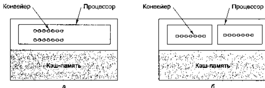
Рис. 8.8. Однокристальные мультипроцессоры: микросхема с двумя конвейерами (а); микросхема с двумя ядрами (б)
