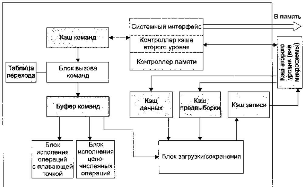
Рис. 4.33. Структурная схема процессора UltraSPARC III Cu
