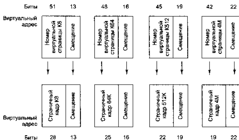
Рис. 6.15. Отображение виртуальных адресов на физические в машине UltraSPARC III
