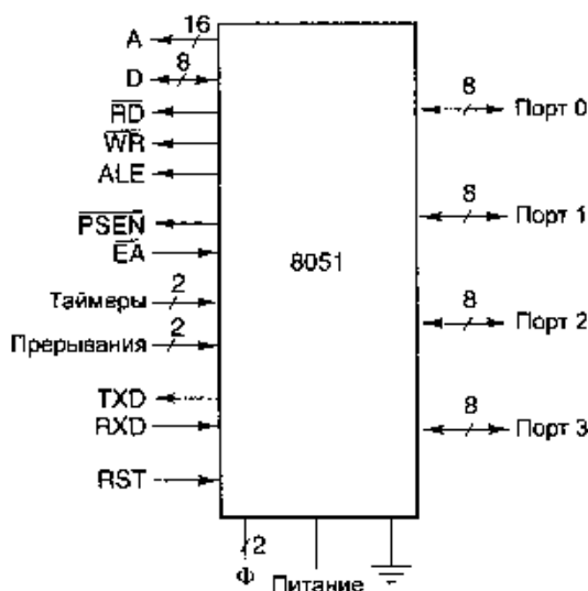
Рис. 3.47. Цоколевка микросхемы 8051
