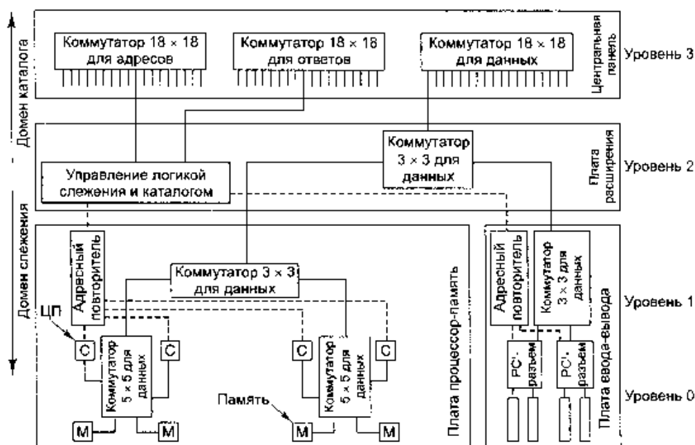
Рис. 8.29. Четырехуровневое соединение блоков в Sun Fire E25K. Пунктирные линии означают передачу адресов, сплошные — передачу данных
