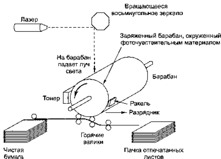
Рис. 2.31. Схема работы лазерного принтера
