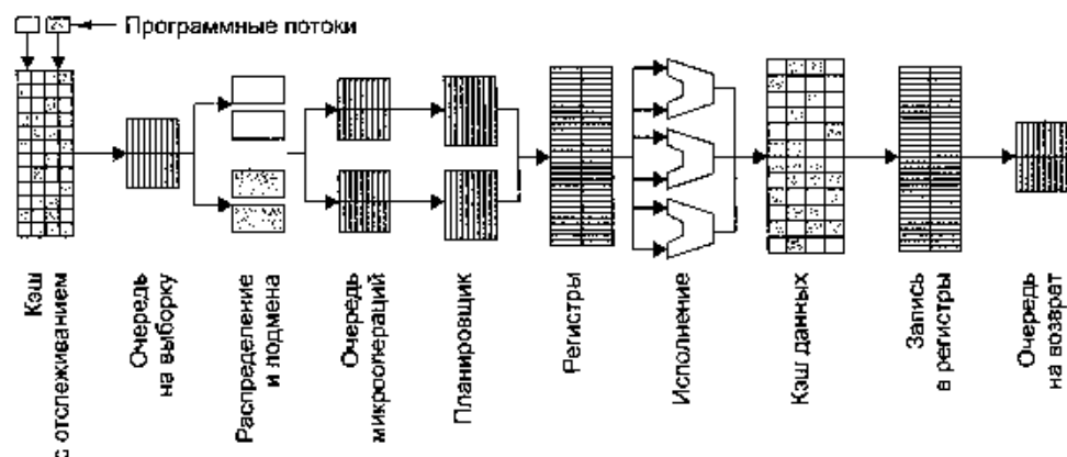
Рис. 8.7. Разделение ресурсов между программными потоками в микроархитектуре NetBurst, реализованной в Pentium 4
