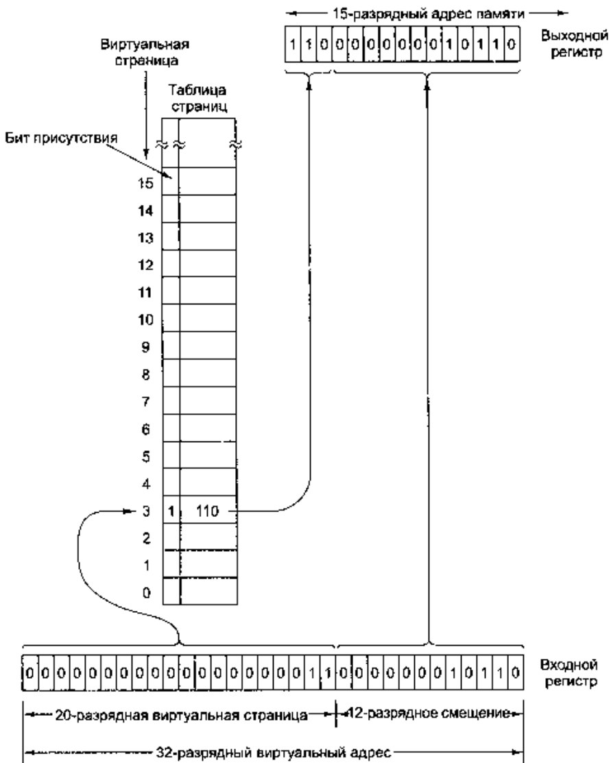
Рис. 6.4. Формирование адреса основной памяти из адреса виртуальной памяти
