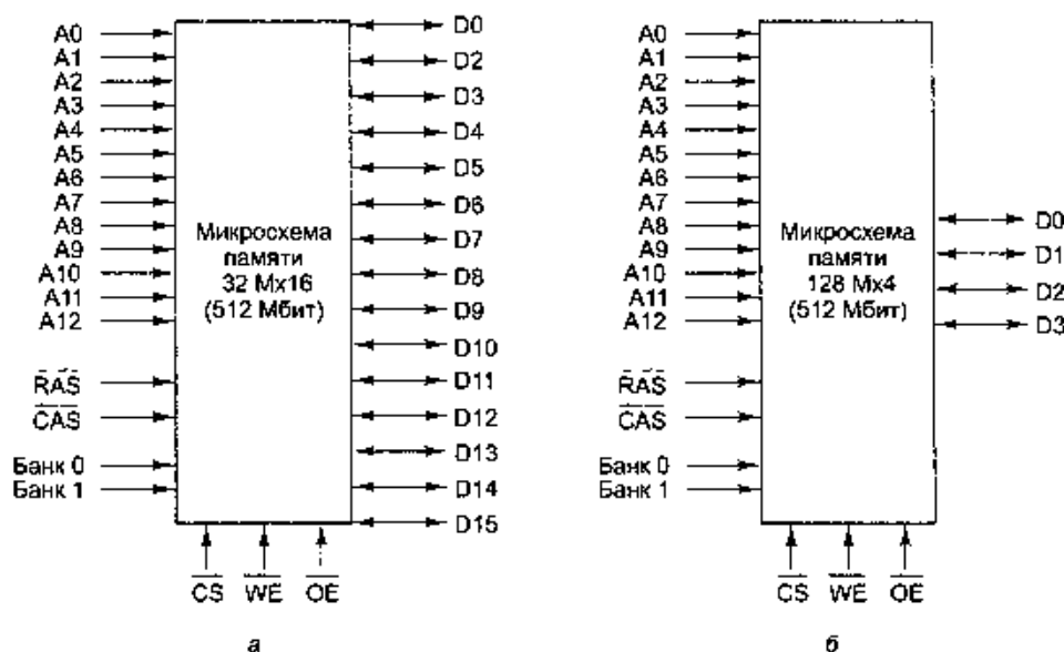
Рис. 3.31. Два способа организации микросхемы памяти объемом 512 Мбит
