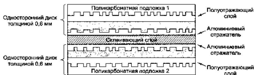
Рис. 2.23. Двухсторонний DVD-диск с двойным слоем
