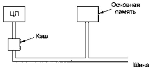
Рис. 2.13. Кэш-память по логике вещей должна находиться между процессором и основной памятью. В действительности существует три возможных варианта размещения кэш-памяти
