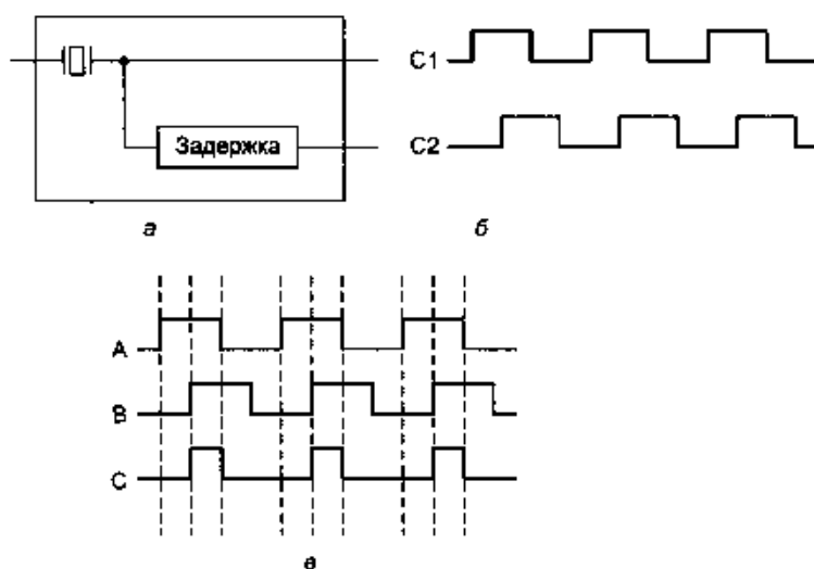
Рис. 3.20. Тактовый генератор (а); временная диаграмма тактового генератора (б); порождение асинхронных тактовых импульсов (в)
