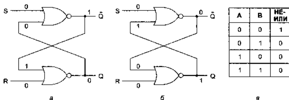
Рис. 3.21. Защелка НЕ-ИЛИ в состоянии 0 (а); защелка НЕ-ИЛИ в состоянии 1 (б); таблица истинности для функции НЕ-ИЛИ (в)
