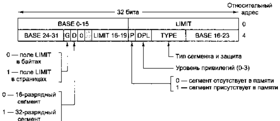
Рис. 6.11. Дескриптор сегмента кода Pentium 4. Сегменты данных практически ничем не различаются
