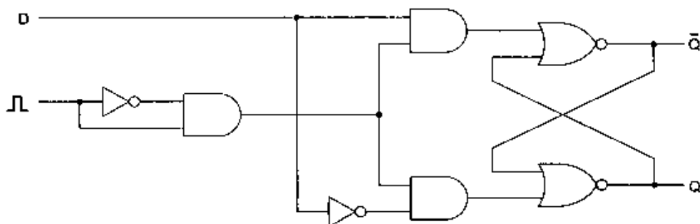
Рис. 3.25. D-триггер
