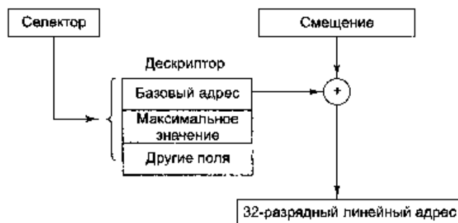
Рис. 6.12. Преобразование пары селектор-смещение в линейный адрес
