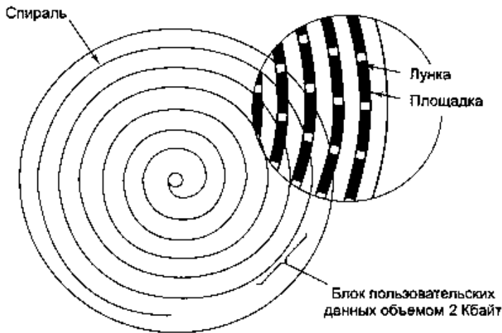
Рис. 2.20. Схема записи компакт-диска
