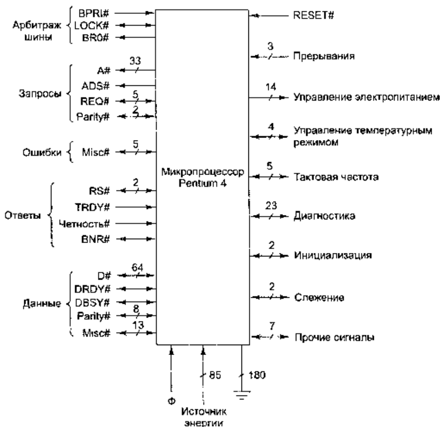
Рис. 3.42. Цоколевка процессора Pentium 4. Официальные названия отдельных сигналов даны прописными буквами; общепринятые названия групп связанных сигналов и описания сигналов — строчными
