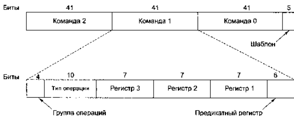
Рис. 5.30. Пучок в архитектуре IA-64 состоит из трех команд
