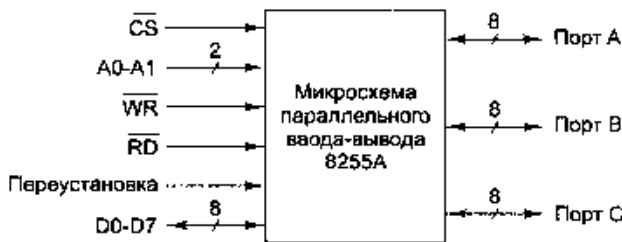
Рис. 3.56. Микросхема 8255A
