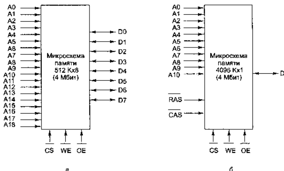
Рис. 3.30. Два способа организации памяти объемом 4 Мбит
