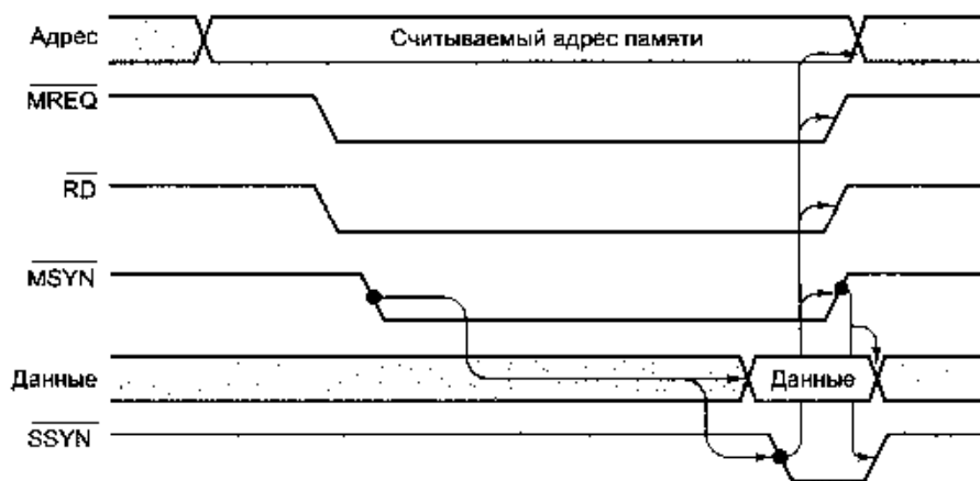
Рис. 3.36. Работа асинхронной шины
