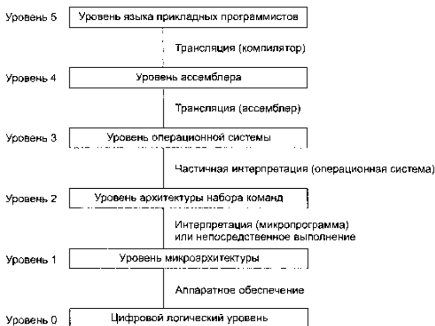
Рис. 1.2. Шестиуровневый компьютер. Способ поддержки каждого уровня указан под ним, в скобках дано название соответствующего программного обеспечения
