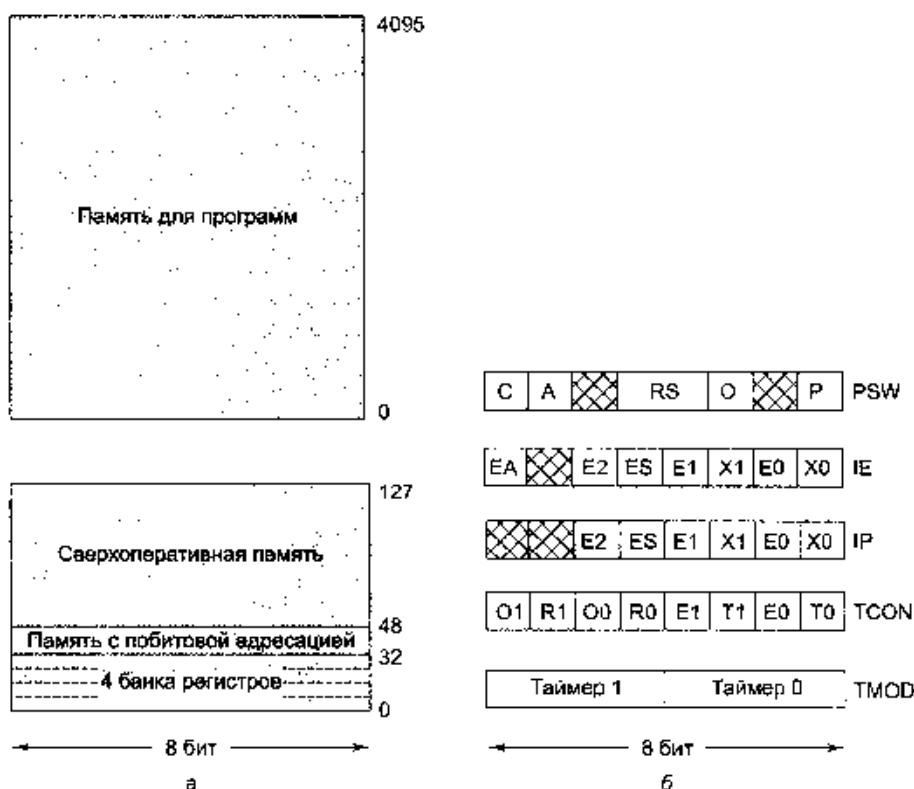
Рис. 5.5. Организация встроенной в микросхему памяти 8051 (а); основные регистры 8051 (б)
