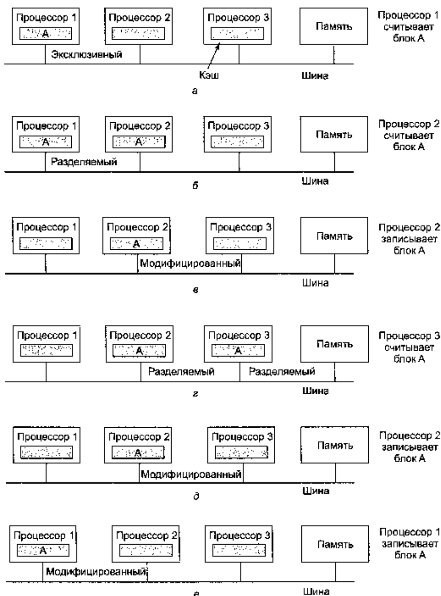
Рис. 8.22. Иллюстрация протокола MESI
