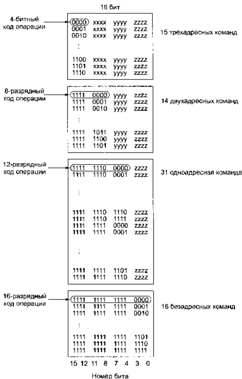
Рис. 5.9. Расширение кода операции обеспечивает 15 трехадресных команд, 14 двухадресных команд, 31 одноадресную команду и 16 безадресных команд. Поля xxxx, yyyy и zzzz — это 4-разрядные адресные поля
