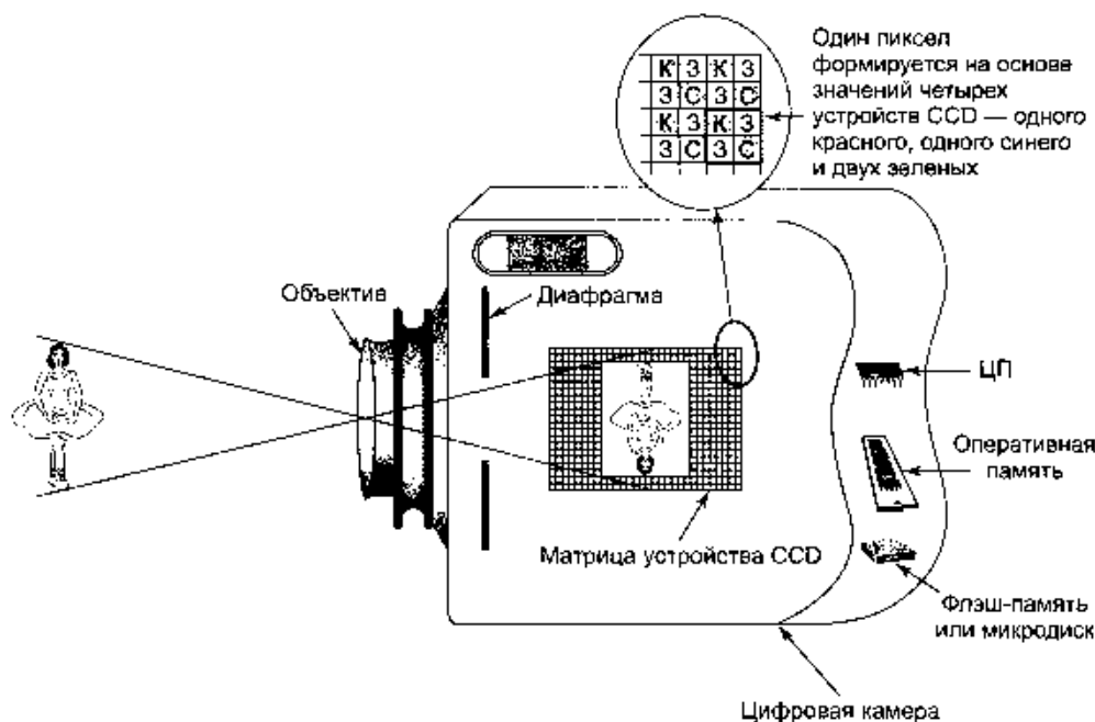
Рис. 2.38. Цифровая камера
