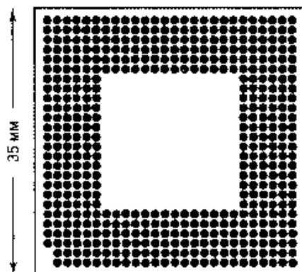
Рис. 3.41. Компоновка Pentium 4
