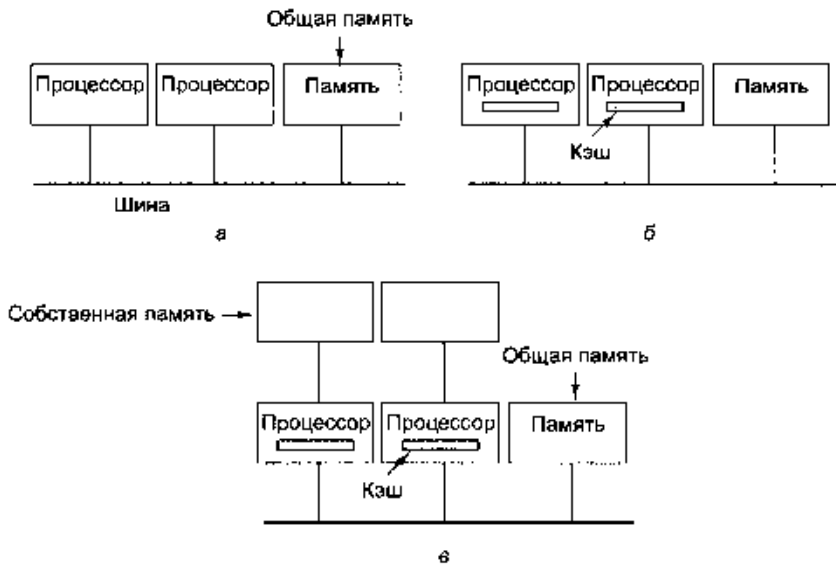
Рис. 8.21. Три варианта мультипроцессора на одной шине: без кэш-памяти (а); с кэш-памятью (б); с кэш-памятью и отдельными модулями локальной памяти (в)
