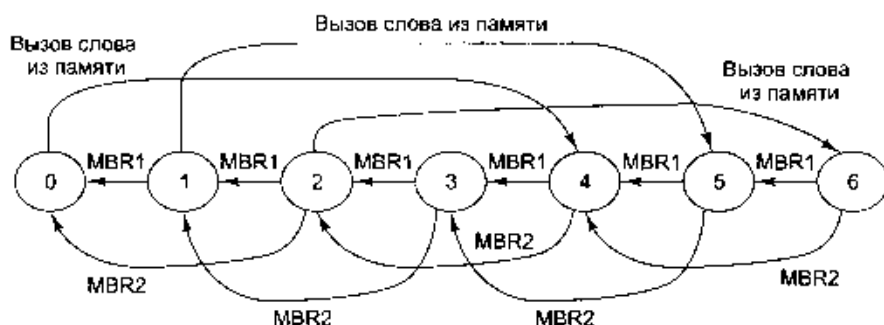
Рис. 4.19. Конечный автомат для реализации блока выборки команд
