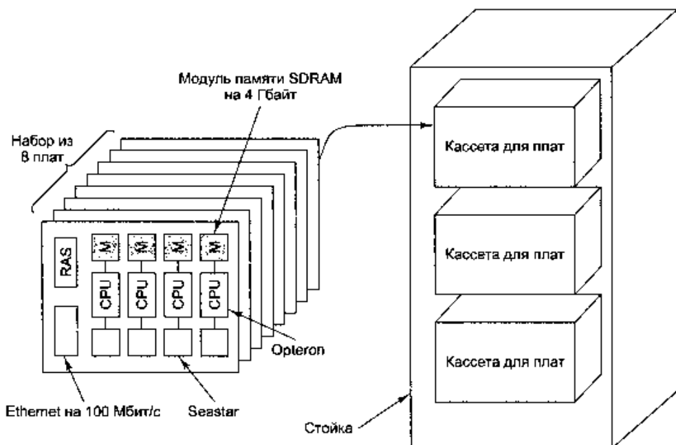
Рис. 8.34. Размещение компонентов Red Storm
