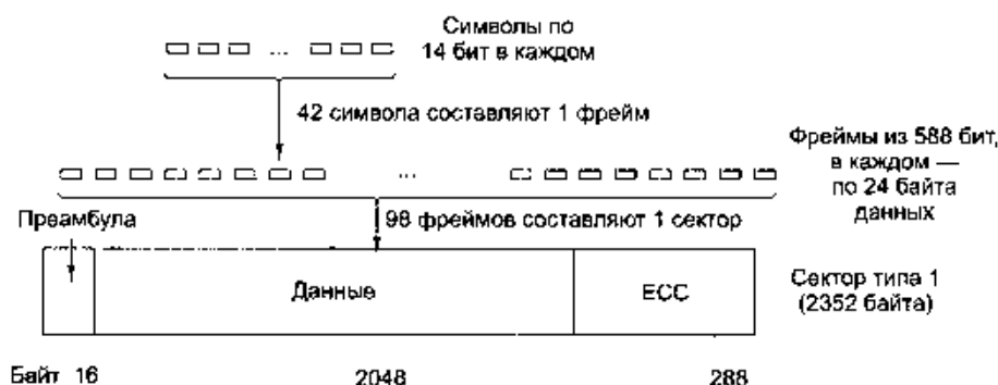
Рис. 2.21. Схема расположения данных на компакт-диске
