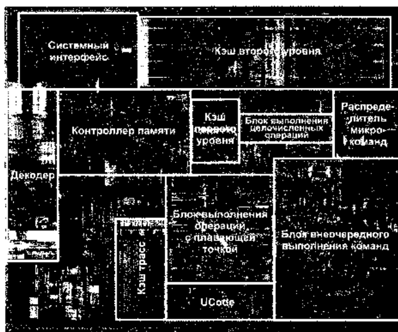
Рис. 1.8. Микросхема Pentium 4 (фотография используется с разрешения корпорации Intel)
