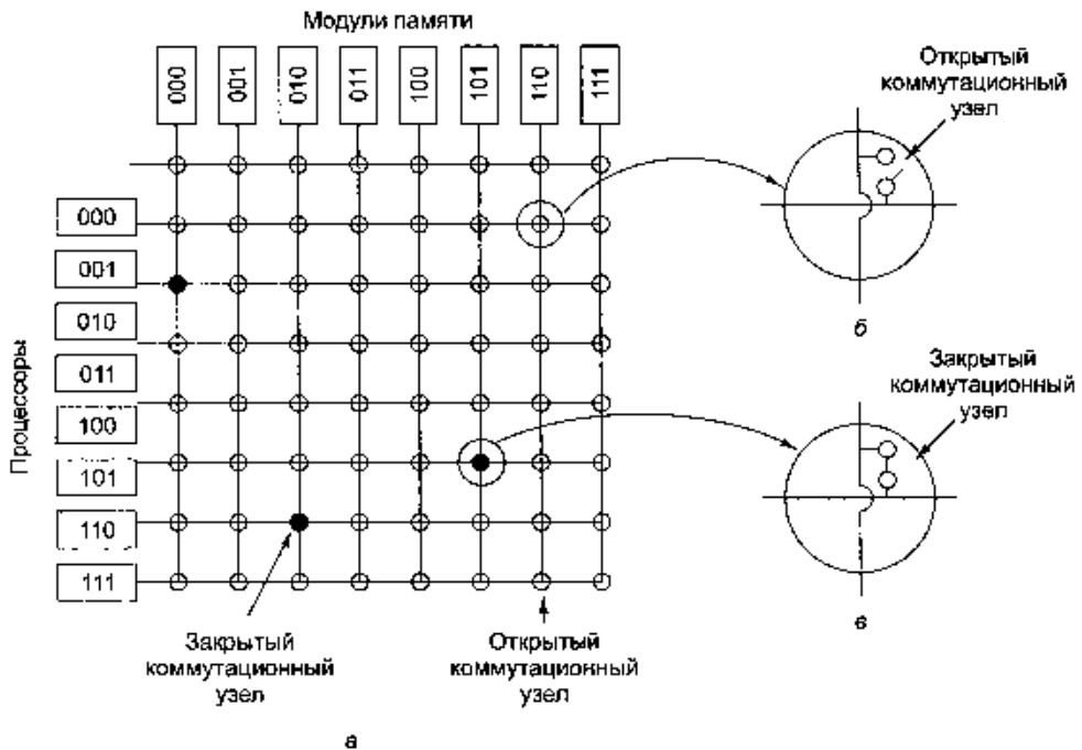
Рис. 8.23. Перекрестная коммутация 8 \times 8 (а); открытый узел (б); закрытый узел (в)
