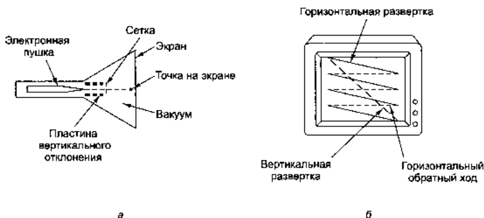
Рис. 2.27. Поперечное сечение электронно-лучевой трубки (а); схема развертки электронно-лучевой трубки (б)
