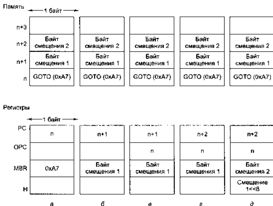
Рис. 4.17. Ситуация в начале выполнения различных микрокоманд: Main1 (а); goto1 (б); goto2 (в); goto3 (г); goto4 (д)
