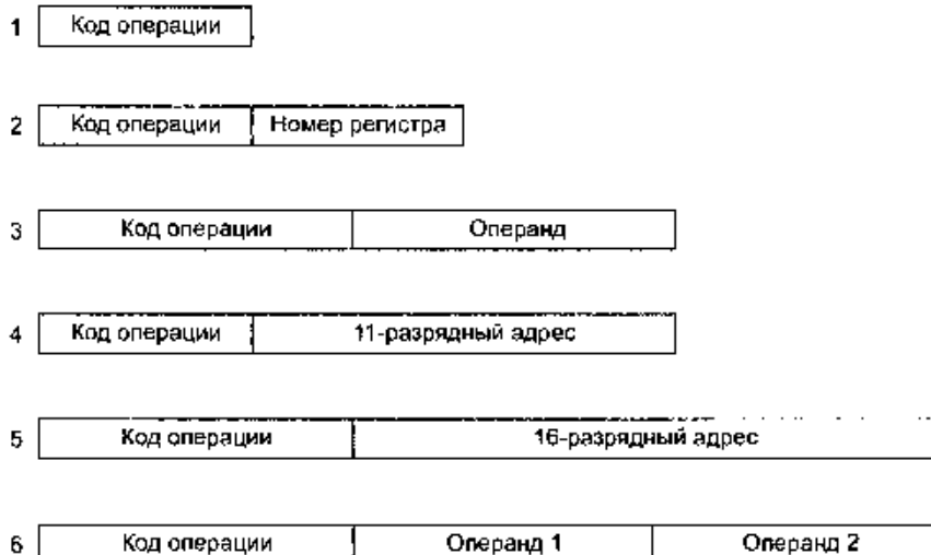
Рис. 5.12. Форматы команд 8051
