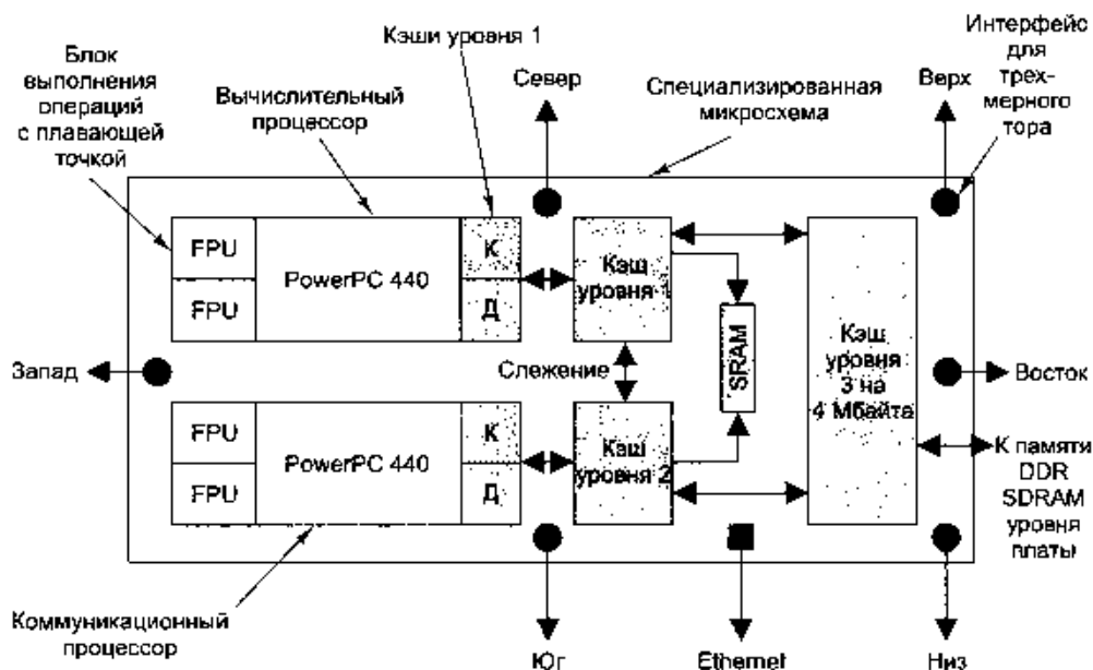
Рис. 8.32. Специализированный микропроцессор в системе BlueGene/L
