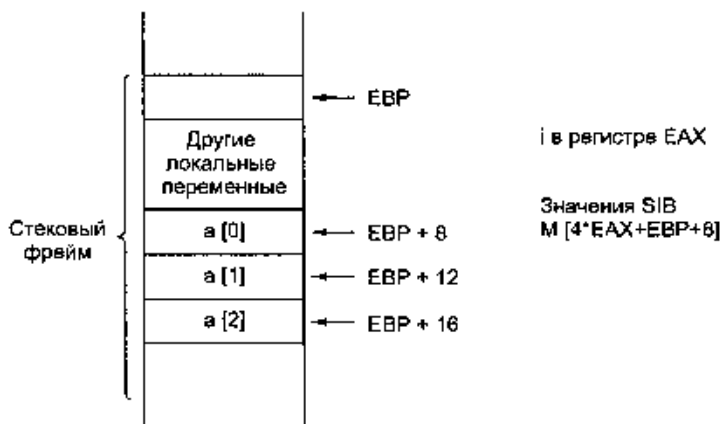
Рис. 5.19. Обращение к элементу массива a[i]
