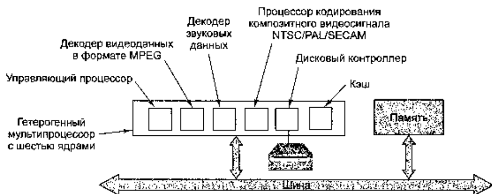
Рис. 8.9. Логическая схема простого DVD-плеера с гетерогенным мультипроцессором и несколькими специализированными ядрами для выполнения различных функций
