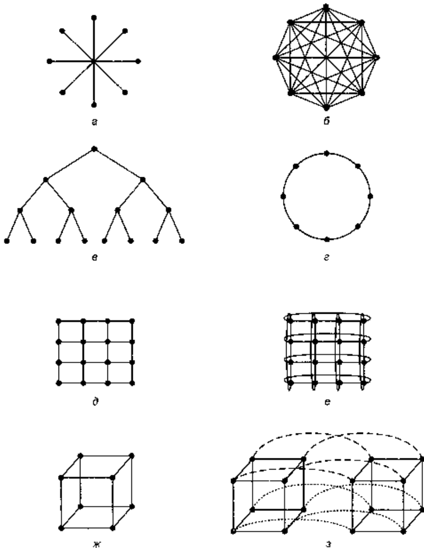
Рис. 8.31. Различные топологии. Жирные точки соответствуют коммутаторам. Процессоры и модули памяти не показаны: звезда (а); полная взаимосвязь (б); дерево (в); кольцо (г); решетка (д); двойной тор (е); куб (ж); четырехмерный гиперкуб (з)
