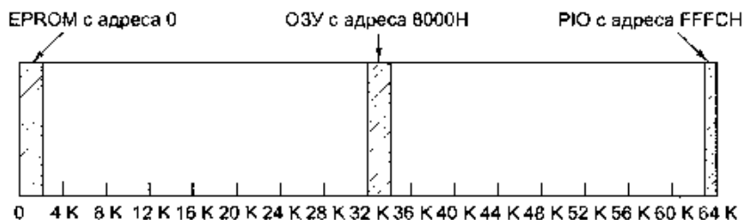
Рис. 3.57. Расположение EPROM, ОЗУ и PIO в пространстве из 64К адресов
