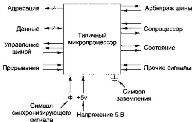
Рис. 3.32. Цоколевка типичного центрального процессора. Стрелочки указывают входные и выходные сигналы. Короткие диагональные линии говорят о наличии нескольких выводов данного типа. Число этих выводов зависит от модели процессора
