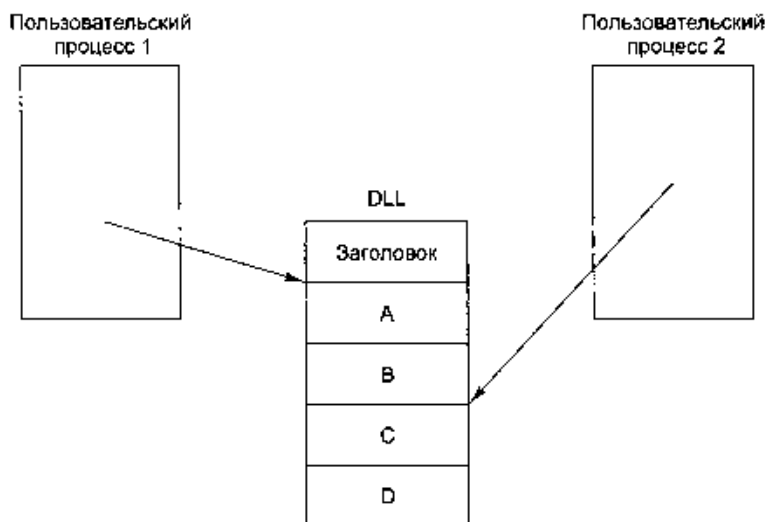
Рис. 7.7. Два процесса используют один DLL-файл
