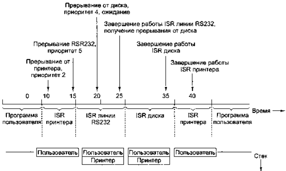
Рис. 5.28. Пример с несколькими прерываниями. Последовательность действий
