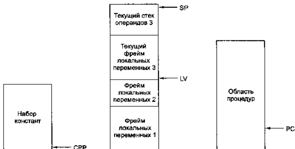
Рис. 4.9. Области памяти IJVM
