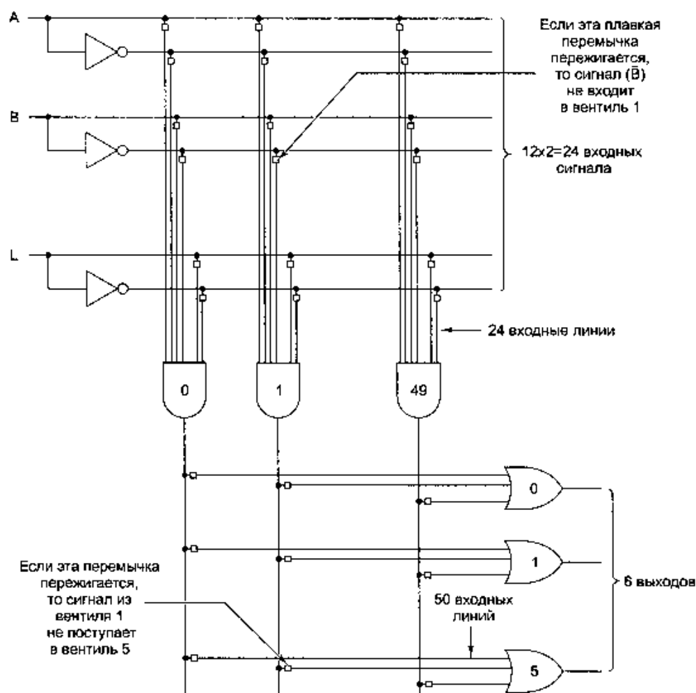
Рис. 3.14. Программируемая логическая матрица с 12 входами и 6 выходами. Маленькие квадратики — плавкие перемычки, выжигаемые для получения нужной функции. Плавкие перемычки упорядочиваются в двух матрицах, верхняя матрица — для вентилях И, нижняя — для вентилях ИЛИ
