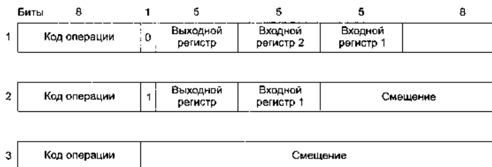
Рис. 5.17. Форматы команд для трехадресной машины
