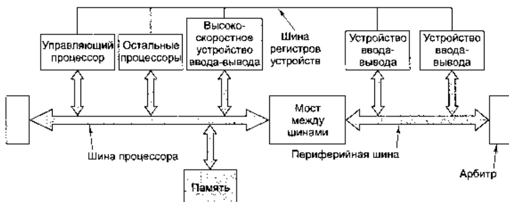
Рис. 8.10. Архитектура CoreConnect компании IBM
