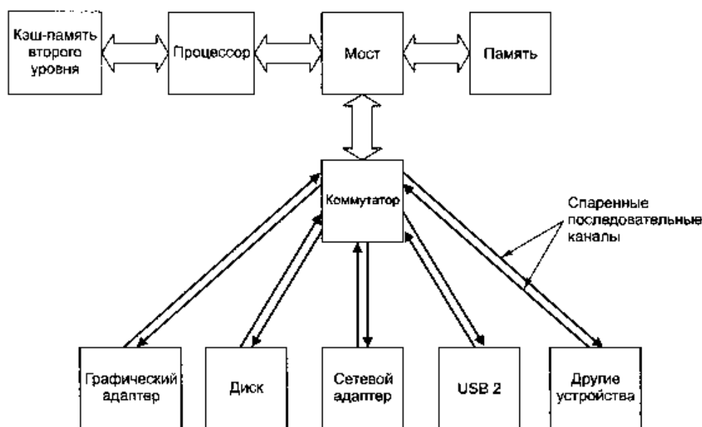
Рис. 3.53. Стандартная компоновка системы PCI Express
