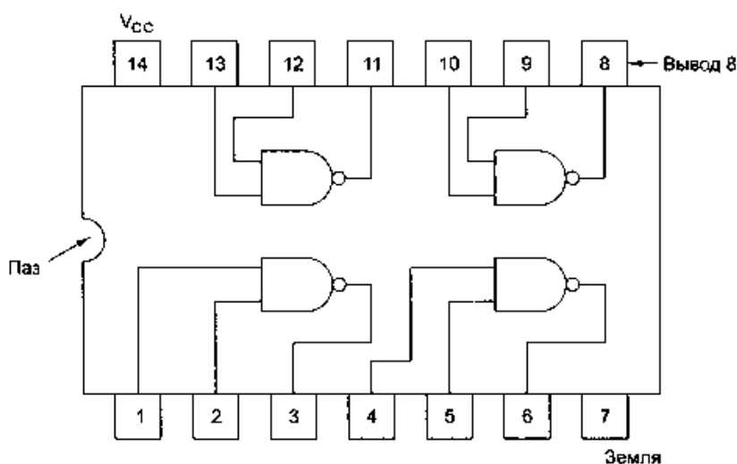
Рис. 3.9. МИС из четырех вентиляей
