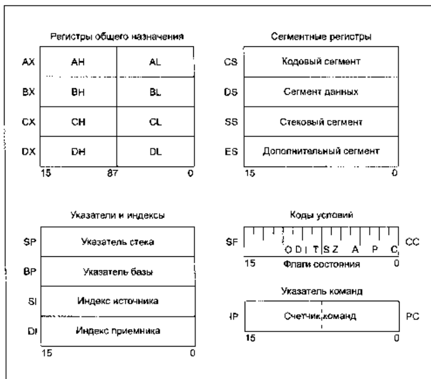
Рис. В.2. Регистры процессора 8088
