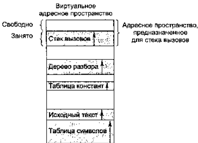
Рис. 6.6. Если в одномерном адресном пространстве размер структур постоянно растет, одна из них может «врезаться» в другую
