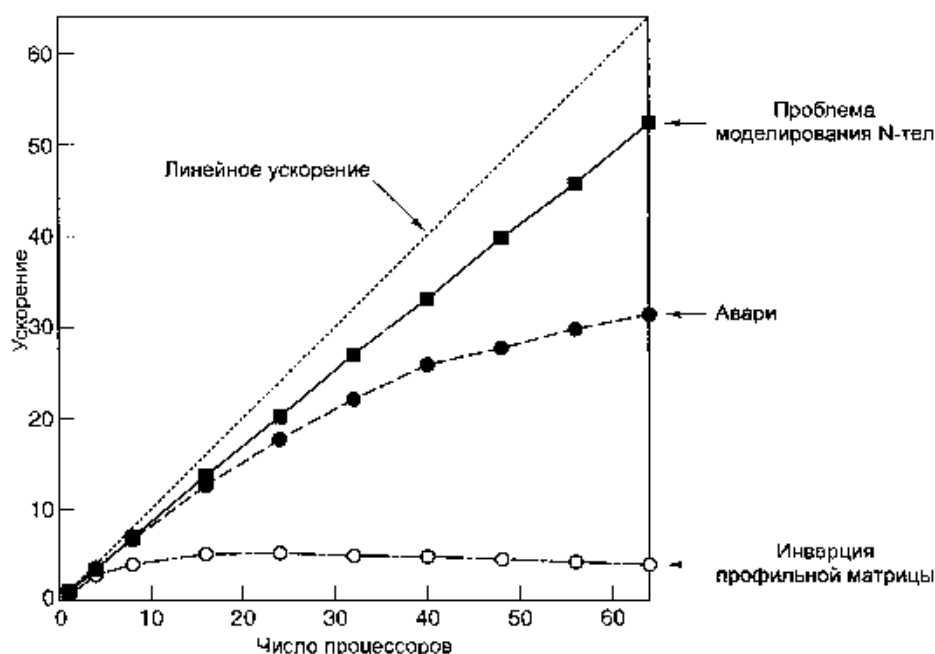
Рис. 8.40. На практике программы не могут достичь идеального ускорения (показано пунктирной линией)
