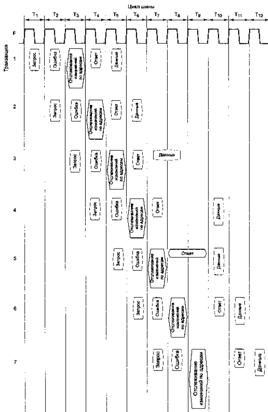
Рис. 3.43. Конвейерный режим шины памяти в системе с процессором Pentium 4
