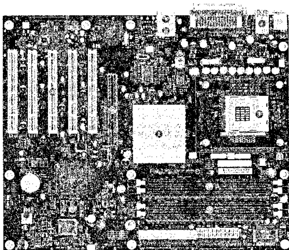
Рис. 1.7. Центральным компонентом любого персонального компьютера является печатная плата. На рисунке изображена системная плата Intel D875PBZ (фотография используется с разрешения корпорации Intel): 1) гнездо для Pentium 4; 2) микросхема поддержки 875P; 3) гнезда для модулей памяти; 4) коннектор AGP; 5) дисковый интерфейс; 6) интерфейс Gigabit Ethernet; 7) пять гнезд PCI; 8) порты USB 2.0; 9) средства охлаждения; 10) BIOS
