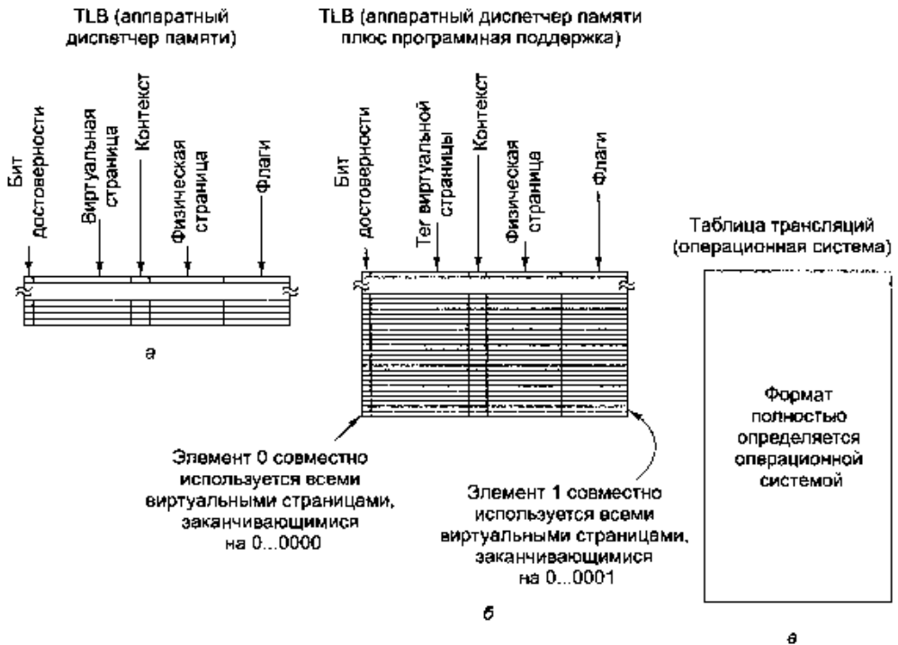
Рис. 6.16. Структуры данных, используемые для трансляции виртуального адреса в машине UltraSPARC III: буфер TLB (а); буфер TSB (б); таблица трансляции (в)
