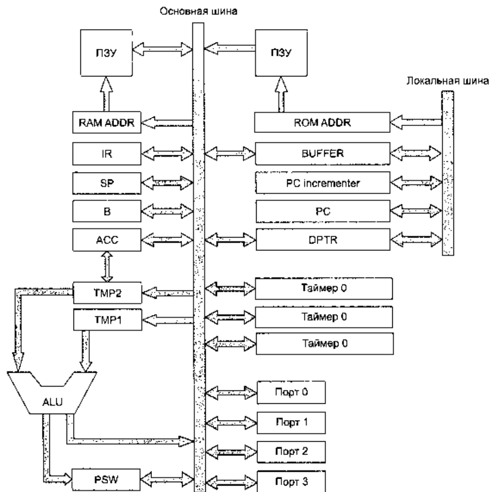
Рис. 4.35. Микроархитектура процессора 8051
