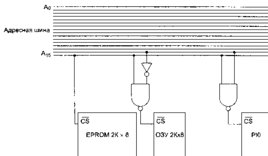
Рис. 3.58. Полное декодирование адреса (а); частичное декодирование адреса (б)
