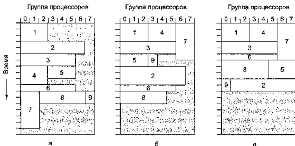
Рис. 8.38. Выполнение заданий в кластере (серым цветом показаны простаивающие процессоры): в порядке FIFO (а); без блокирования начала очереди (б); путем заполнения прямоугольника в системе координат процессоры — время (в)
