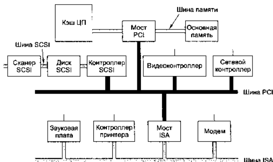
Рис. 2.26. Современный персональный компьютер с шинами PCI и ISA. Модем и звуковая карта относятся к ISA-устройствам, контроллер SCSI является PCI-устройством
