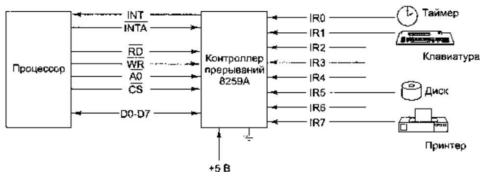
Рис. 3.40. Контроллер прерываний 8259A
