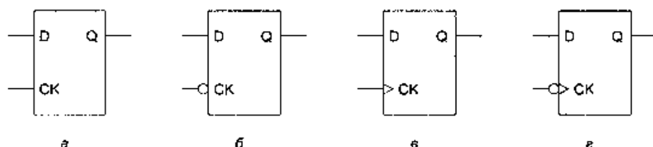
Рис. 3.26. D-защелки и D-триггеры
