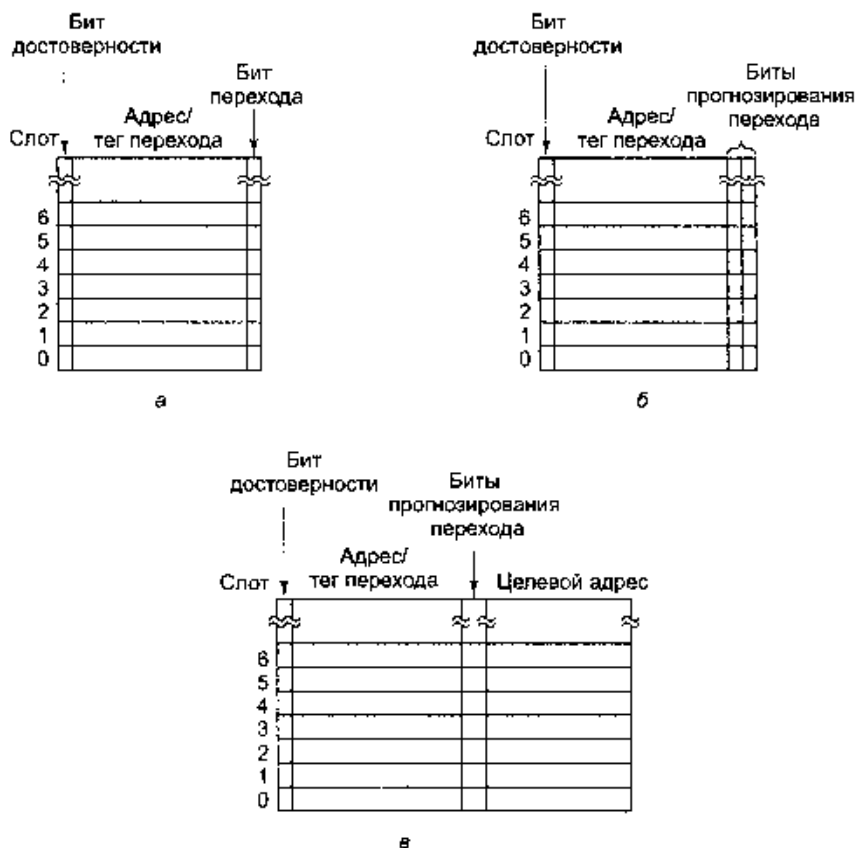
Рис. 4.28. Таблица динамики ветвлений с одnorазрядным указателем перехода (а); таблица динамики ветвлений с 2-разрядным указателем перехода (б); соответствие между адресом команды перехода и целевым адресом (в)
