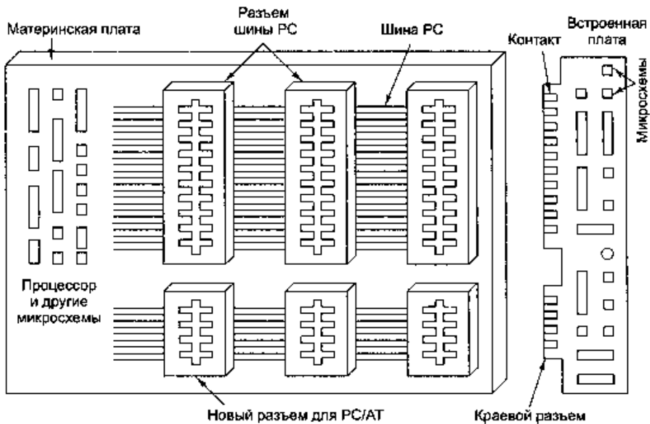
Рис. 3.48. Шина PC/AT объединяет старую и новую шины
