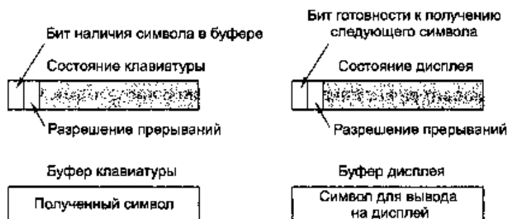
Рис. 5.20. Регистры устройств в простом терминале
