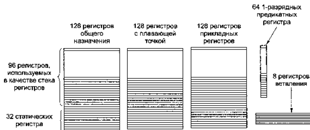
Рис. 5.29. Регистры Itanium 2
