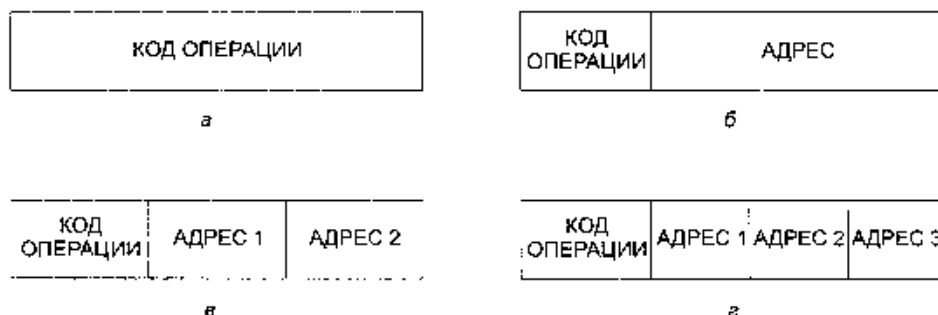
Рис. 5.6. Четыре формата команд: безадресная команда (а); одноадресная команда (б); двухадресная команда (в); трехадресная команда (г)
