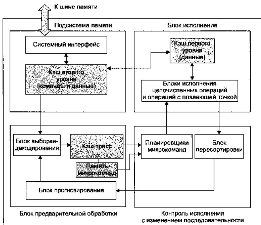
Рис. 4.31. Микроархитектура Pentium 4
