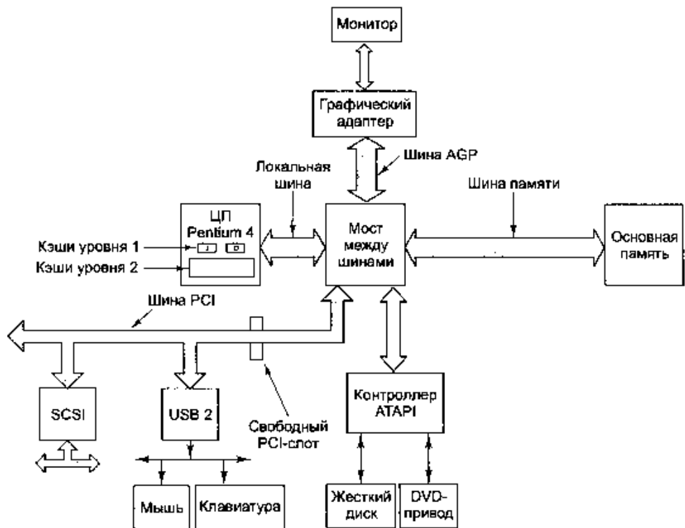
Рис. 3.50. Компоновка шин в современной системе Pentium 4
