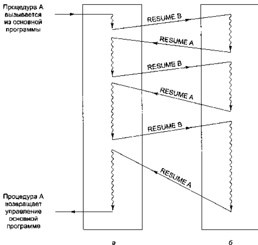
Рис. 5.27. После завершения подпрограммы выполнение начинается с того места, на котором оно завершилось в прошлый раз, а не с самого начала
