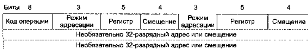
Рис. 5.18. Простые форматы команд для двухадресной машины
