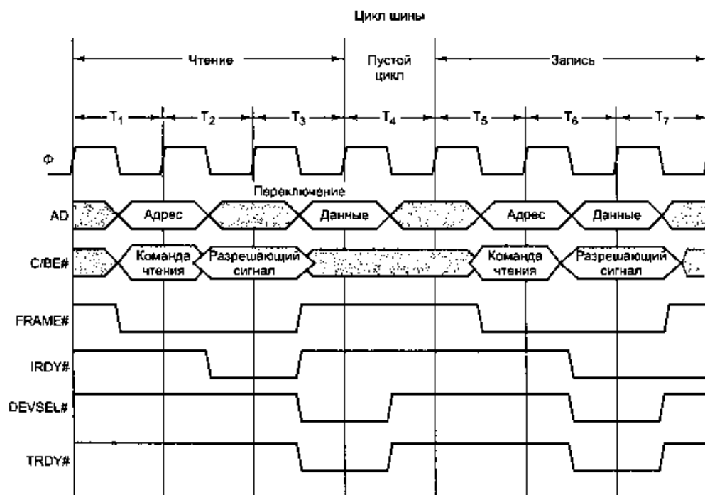
Рис. 3.52. Примеры 32-разрядных транзакций на шине PCI. Во время первых трех циклов происходит операция чтения, затем идет пустой цикл, а следующие три цикла — операция записи
