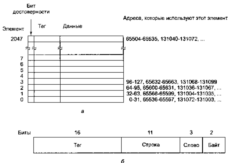
Рис. 4.26. Кэш-память прямого отображения (а); 32-разрядный виртуальный адрес (б)
