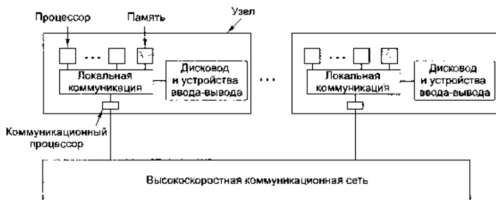
Рис. 8.30. Схема мультикомпьютера
