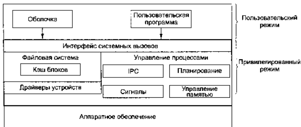
Рис. 6.24. Структура типичной системы UNIX
