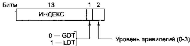
Рис. 6.10. Селектор Pentium 4
