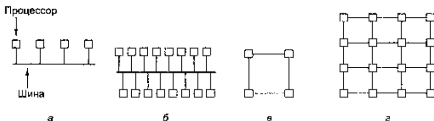
Рис. 8.42. Система из 4 процессоров, связанных общей шиной (а); система из 16 процессоров, связанных общей шиной (б); коммуникационная решетка из 4 процессоров (в); коммуникационная решетка из 16 процессоров (г)
