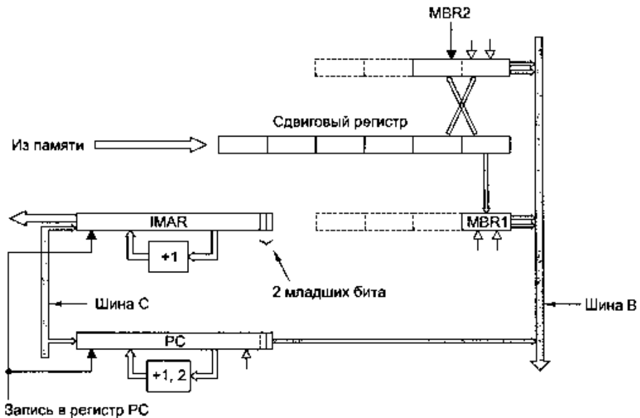
Рис. 4.18. Блок выборки команд в микроархитектуре Mic-1
