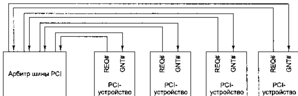
Рис. 3.51. У шины PCI имеется централизованный арбитр
