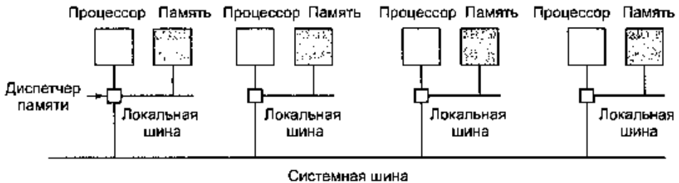
Рис. 8.26. NUMA-машина с двумя уровнями шин
