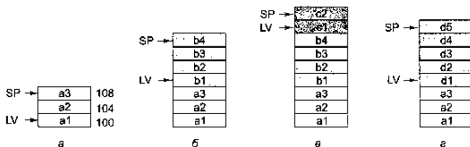
Рис. 4.7. Стек для хранения локальных переменных: во время вызова процедуры A (а); после того, как процедура A вызывает процедуру B (б); после того, как процедура B вызывает процедуру C (в); после того как процедуры C и B завершаются, а процедура A вызывает процедуру D (г)
