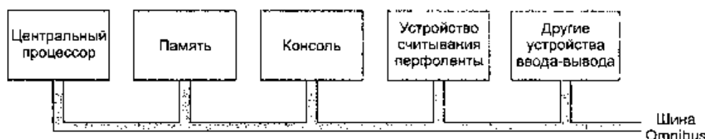
Рис. 1.5. Шина компьютера PDP-8
