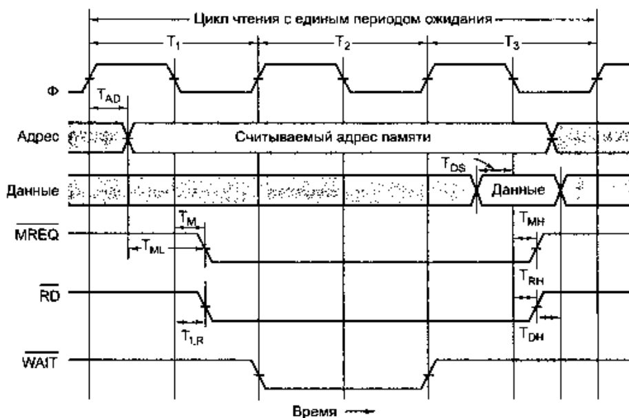
Рис. 3.35. Временная диаграмма процесса считывания на синхронной шине
