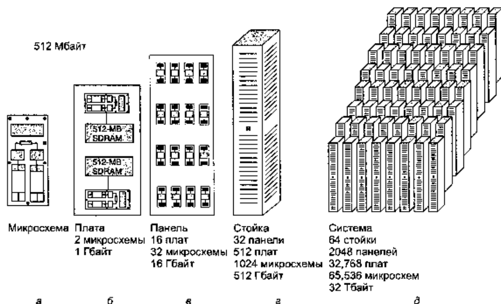
Рис. 8.33. BlueGene/L: микросхема (а), плата (б), панель (в), стойка (г), система (д)
