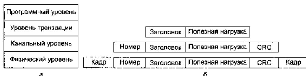
Рис. 3.54. Стек протоколов PCI Express (а); формат пакета (б)
