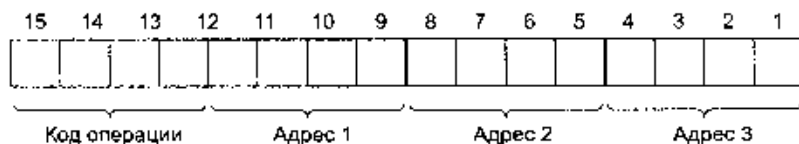
Рис. 5.8. Команда с 4-разрядным кодом операции и тремя 4-разрядными адресными полями
