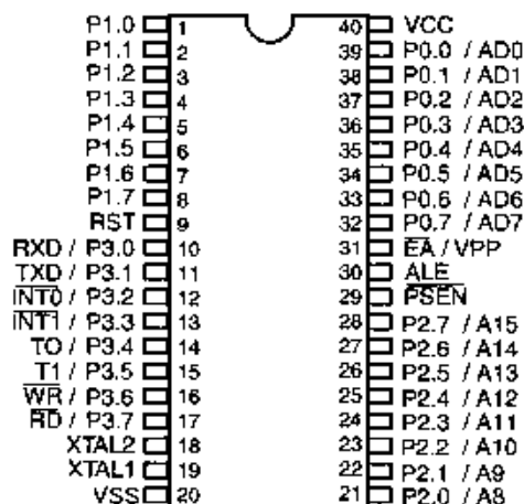
Рис. 3.46. Физическая компоновка микросхемы 8051
