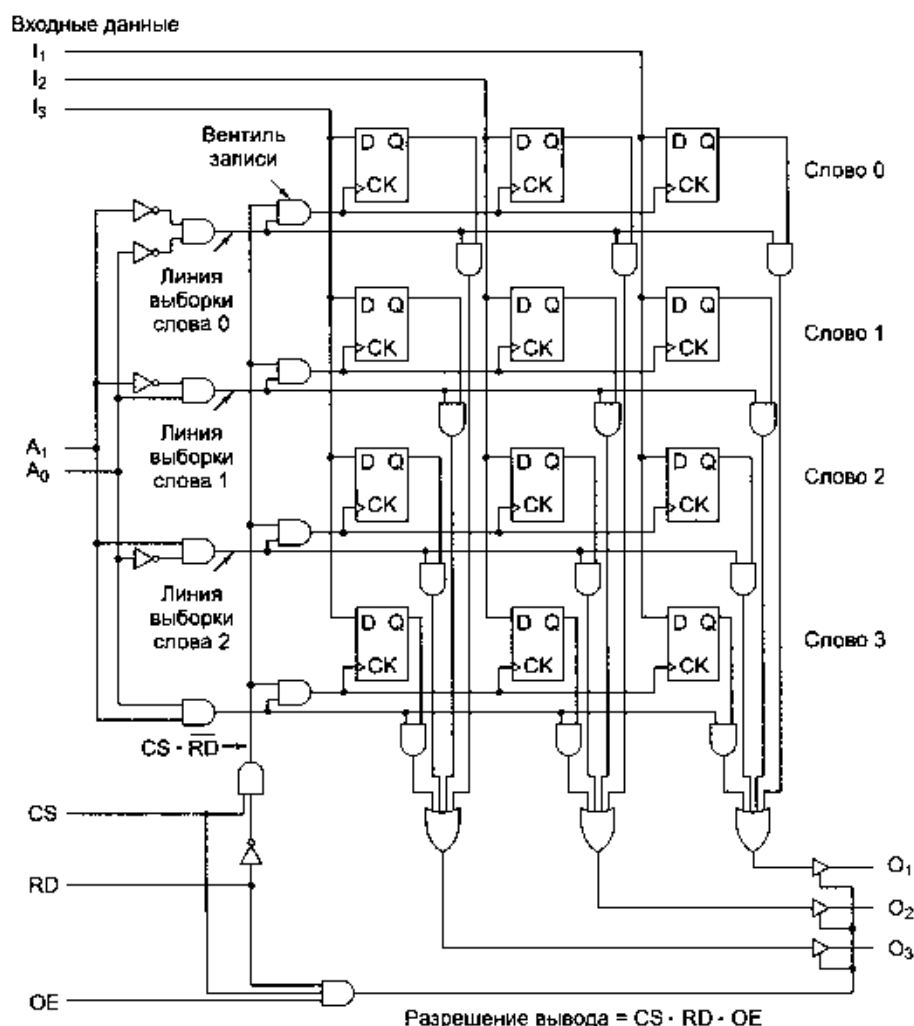
Рис. 3.28. Логическая блок-схема для памяти 4 \times 3 . Каждый ряд представляет одно из 3-разрядных слов. При считывании и записи всегда считывается или записывается целое слово
