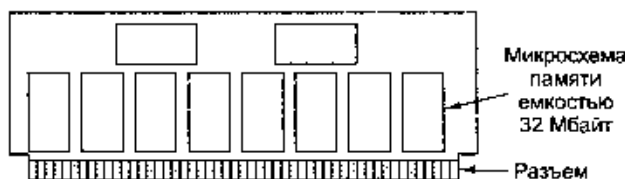
Рис. 2.14. Модуль SIMM объемом 256 Мбайт. Модулем управляют две микросхемы
