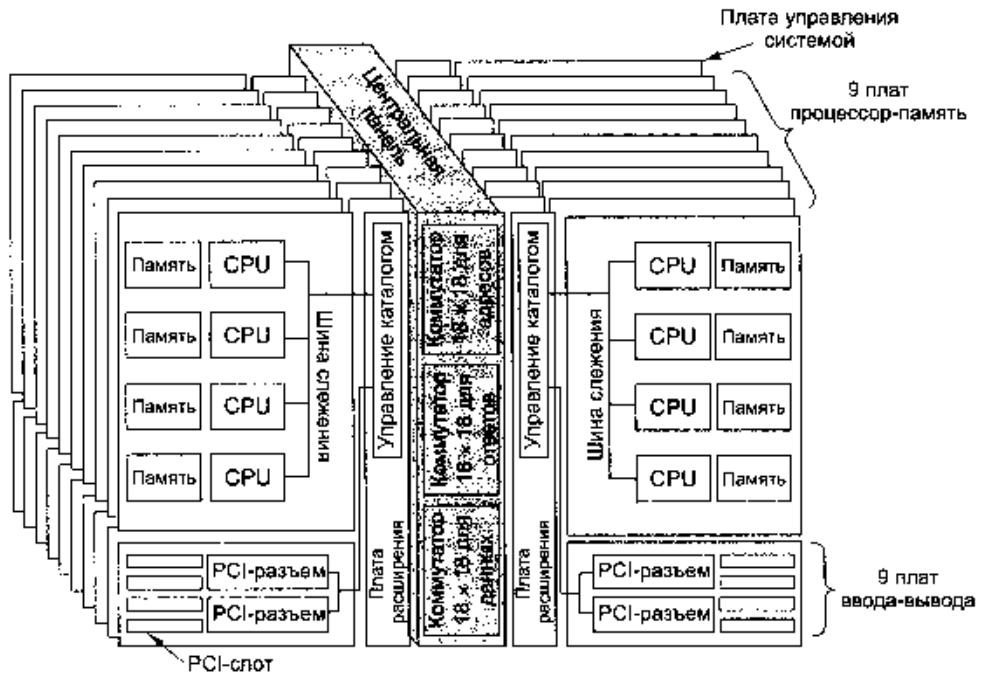
Рис. 8.28. Мультипроцессор E25K компании Sun Microsystems
