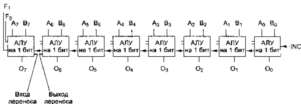
Рис. 3.19. Восемь одноразрядных секций, соединенных в 8-разрядное АЛУ. Для упрощения схемы сигналы разрешения и инверсии не показаны
