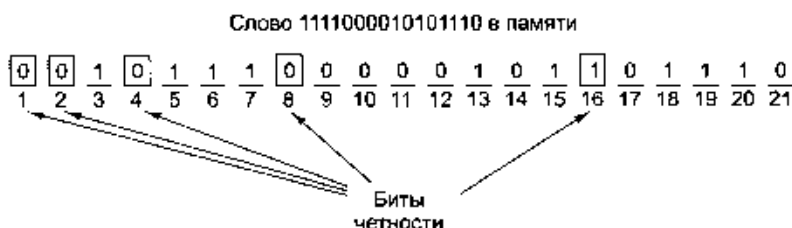
Рис. 2.12. Построение кода Хэмминга для слова 1111000010101110 добавлением к битам данных пяти контрольных разрядов
