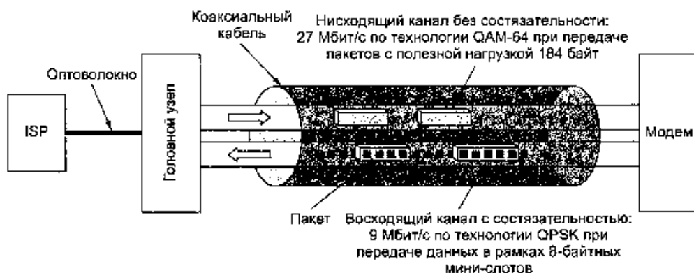
Рис. 2.37. Стандартная организация восходящих и нисходящих каналов в США. Технология QAM-64 (квадратурная амплитудная модуляция) допускает передачу со скоростью 6 бит/Гц, но работает только на высоких частотах. Технология QPSK (квадратурная фазовая модуляция) действует на низких частотах, зато максимальная скорость передачи составляет 2 бит/Гц
