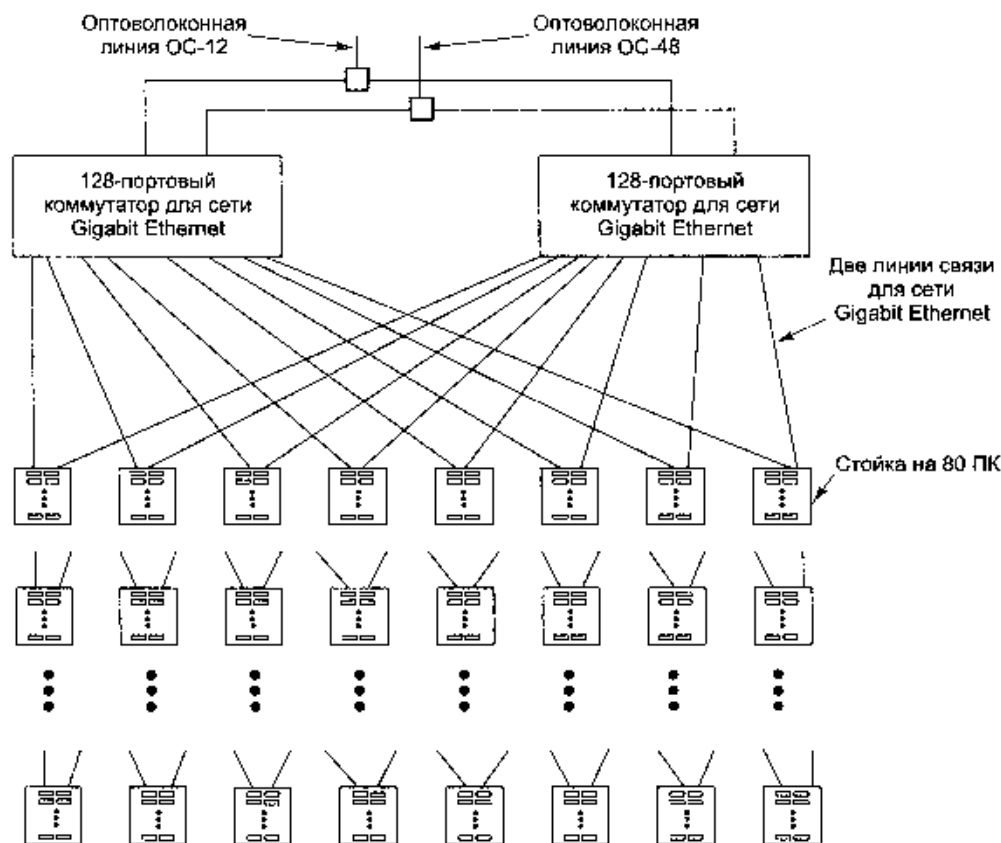
Рис. 8.37. Типичный кластер Google
