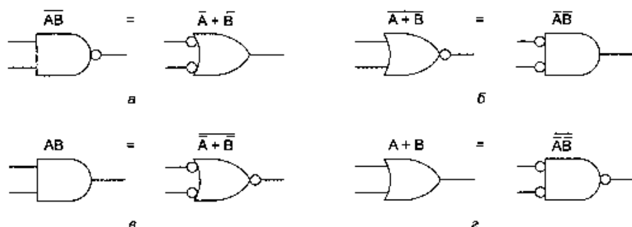
Рис. 3.6. Альтернативные представления некоторых вентилях: НЕ-И (а); НЕ-ИЛИ (б); И (в); ИЛИ (г)
