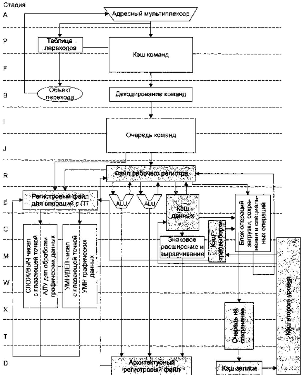
Рис. 4.34. Упрощенная схема конвейера UltraSPARC III Cu
