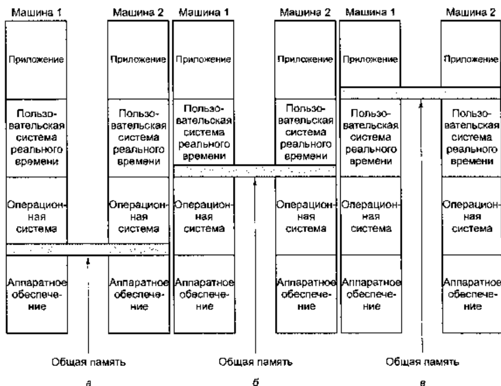
Рис. 8.17. Уровни, на которых можно реализовать общую память: аппаратная реализация (а); операционная система (б); программная реализация (в)
