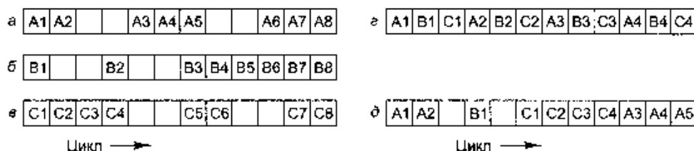
Рис. 8.5. Три программных потока. Пустые квадраты означают простои в ожидании данных из памяти (а–в); мелкомодульная многопоточность (г); крупномодульная многопоточность (д)
