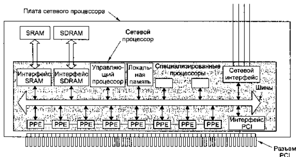
Рис. 8.13. Кристалл и плата типичного сетевого процессора
