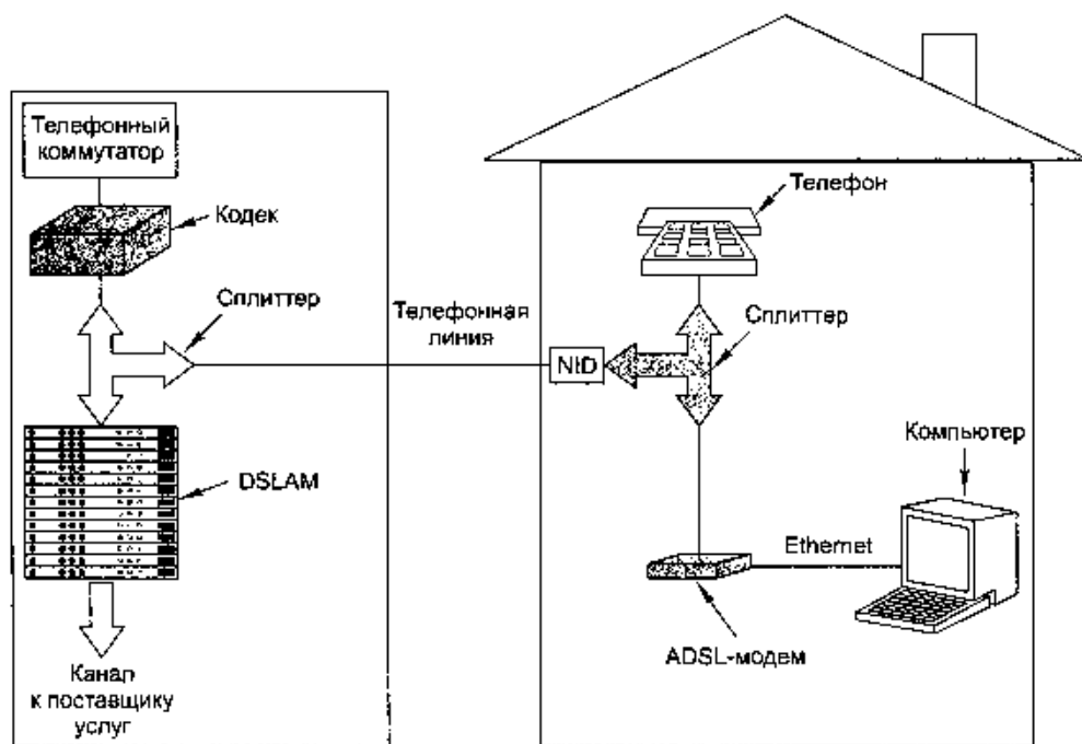
Рис. 2.35. Стандартная конфигурация оборудования ADSL
