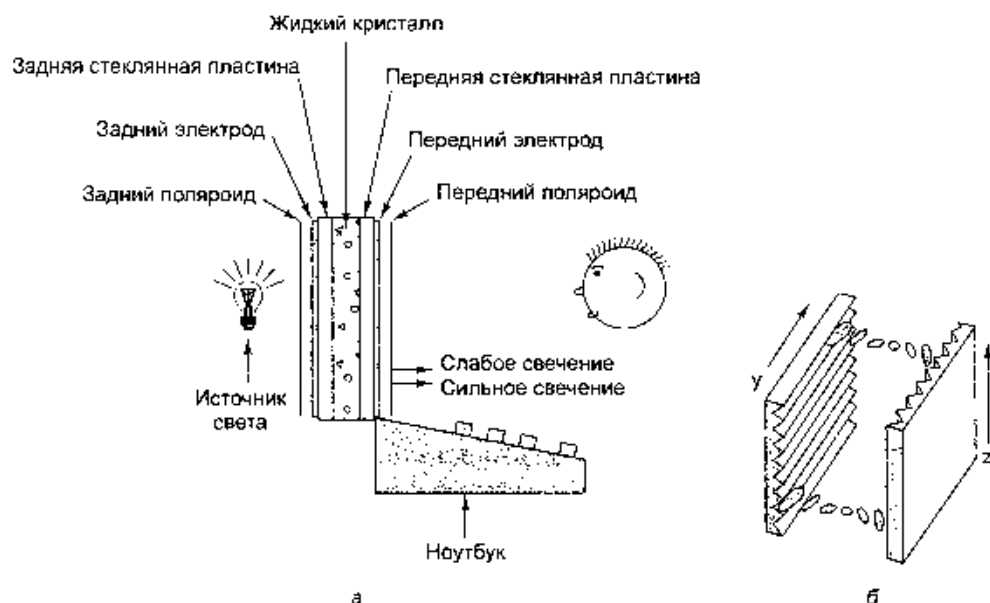
Рис. 2.28. Структура экрана на жидких кристаллах (а); желобки на передней и задней пластинах, расположенные перпендикулярно друг к другу (б)
