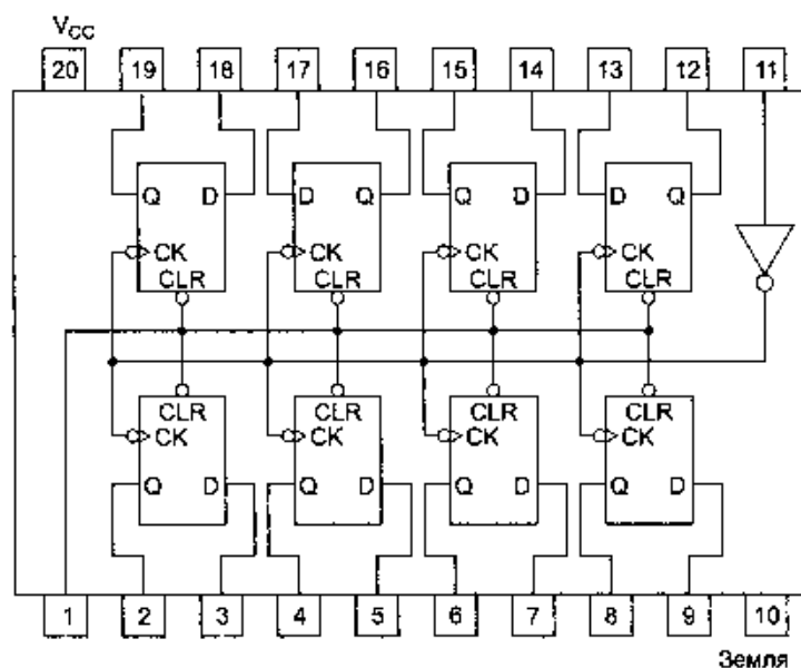
Рис. 3.27. Сдвоенный D-триггер (а), «восьмикратный» триггер (б)
