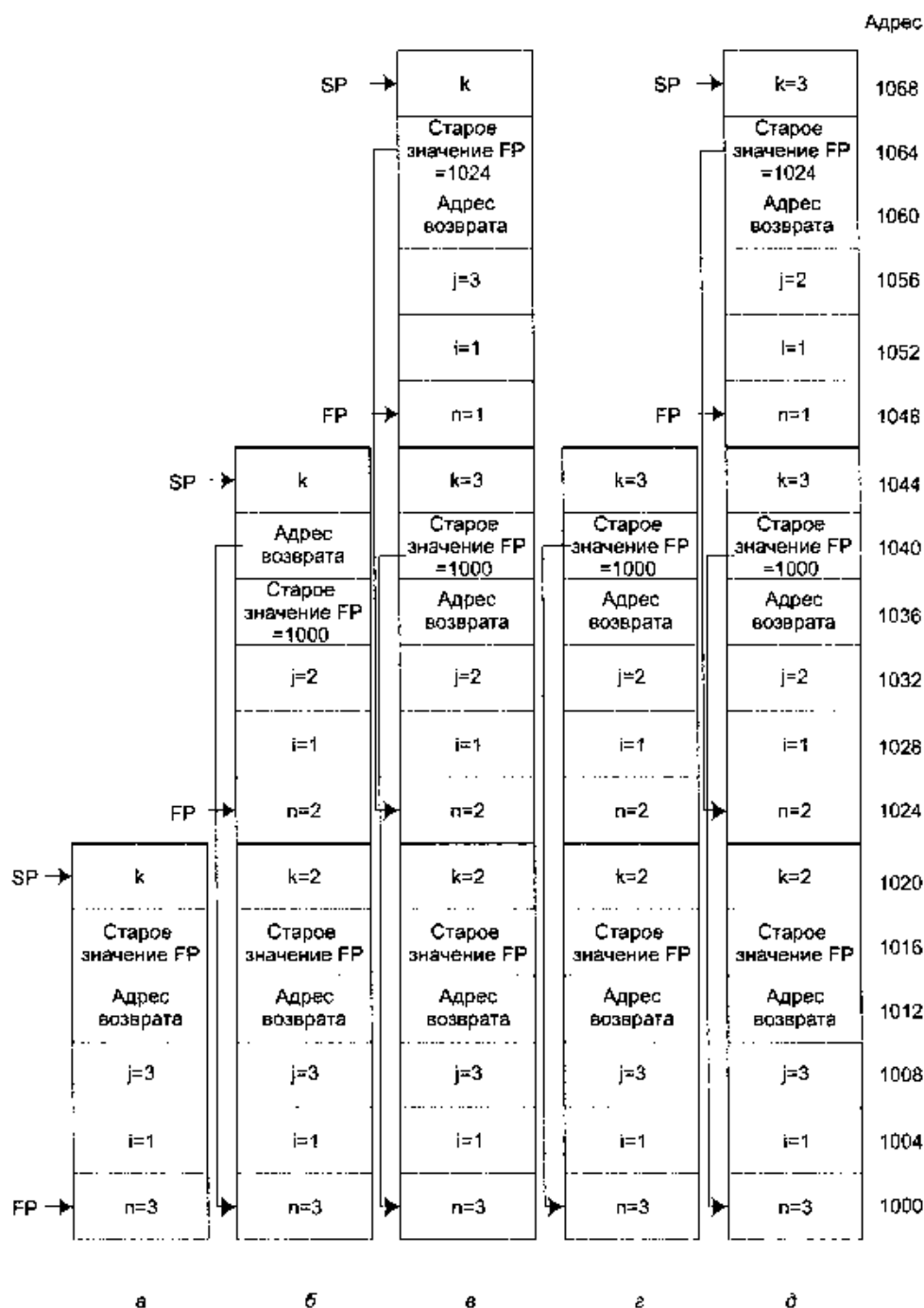
Рис. 5.25. Состояние стека во время выполнения программы из листинга 5.6
