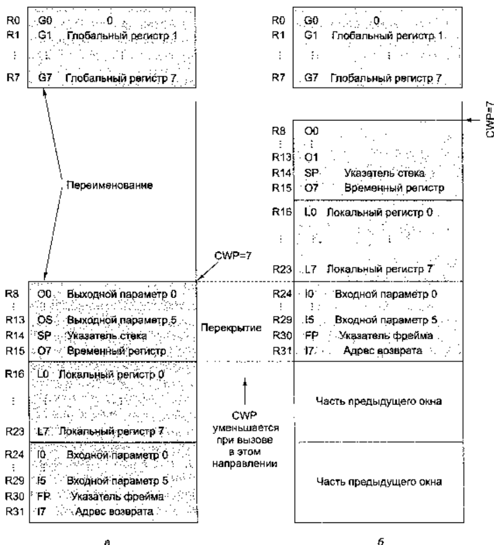
Рис. 5.4. Регистровые окна системы UltraSPARC III
