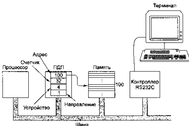
Рис. 5.21. Система с контроллером прямого доступа к памяти
