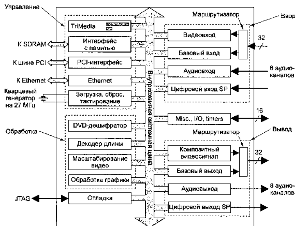
Рис. 8.14. Гетерогенный однокристальный мультипроцессор Nexiperia
