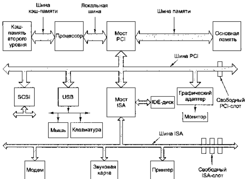
Рис. 3.49. Архитектура типичной системы первых поколений Pentium. (Толщина линий, обозначающих шину, призвана показать ее пропускную способность. Чем толще линия, тем пропускная способность выше.)
