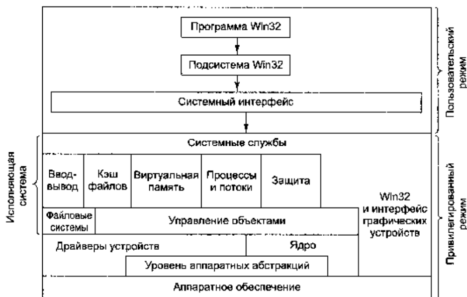
Рис. 6.25. Структура Windows XP
