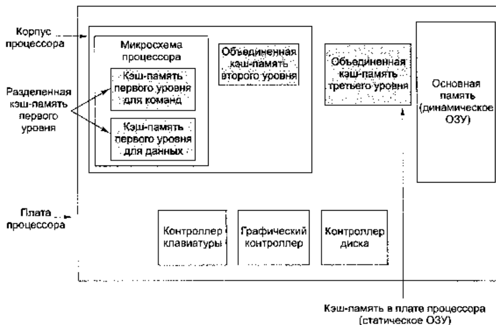
Рис. 4.25. Система с тремя уровнями кэш-памяти
