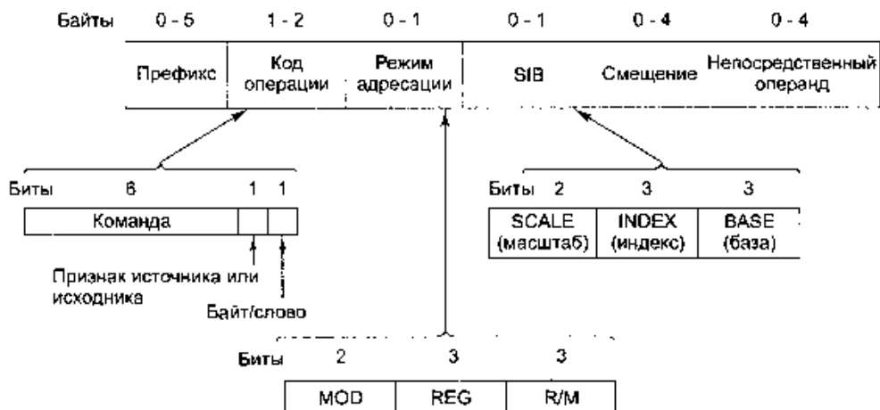
Рис. 5.10. Форматы команд процессора Pentium 4
