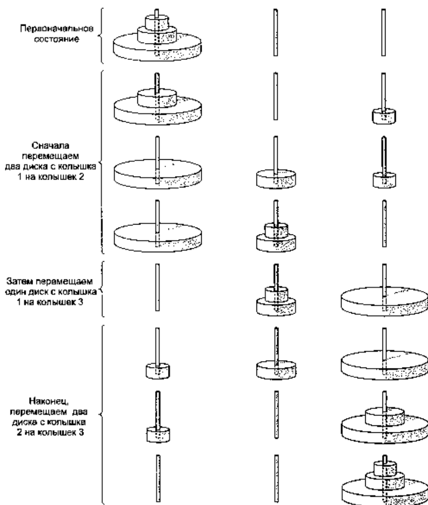
Рис. 5.24. Решение задачи «Ханойская башня» для трех дисков
