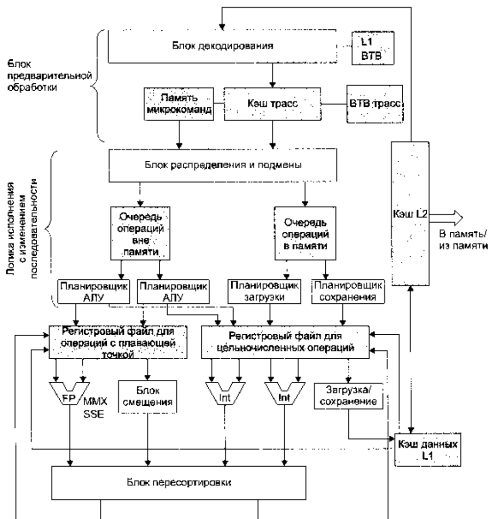
Рис. 4.32. Упрощенная схема тракта данных Pentium 4
