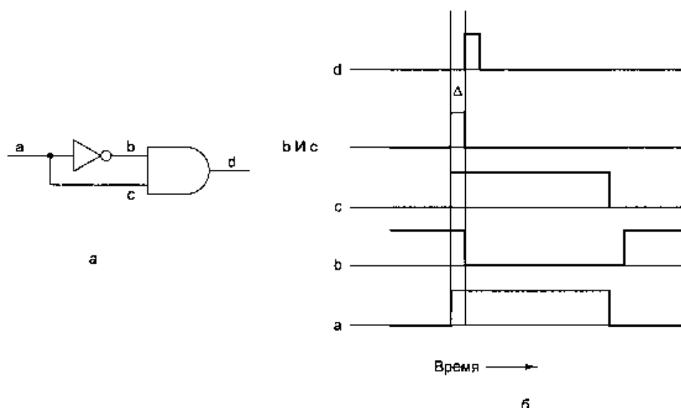
Рис. 3.24. Генератор импульса (а); временная диаграмма для четырех точек на схеме (б)
