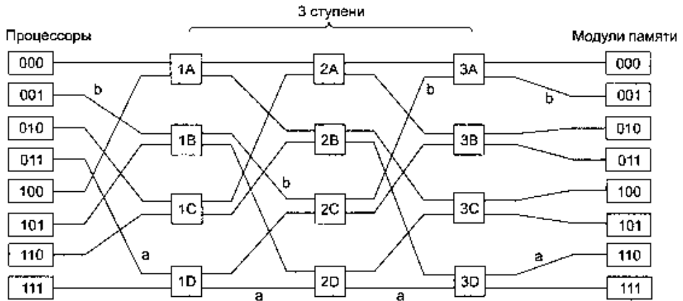
Рис. 8.25. Сеть с многоступенчатой коммутацией омега
