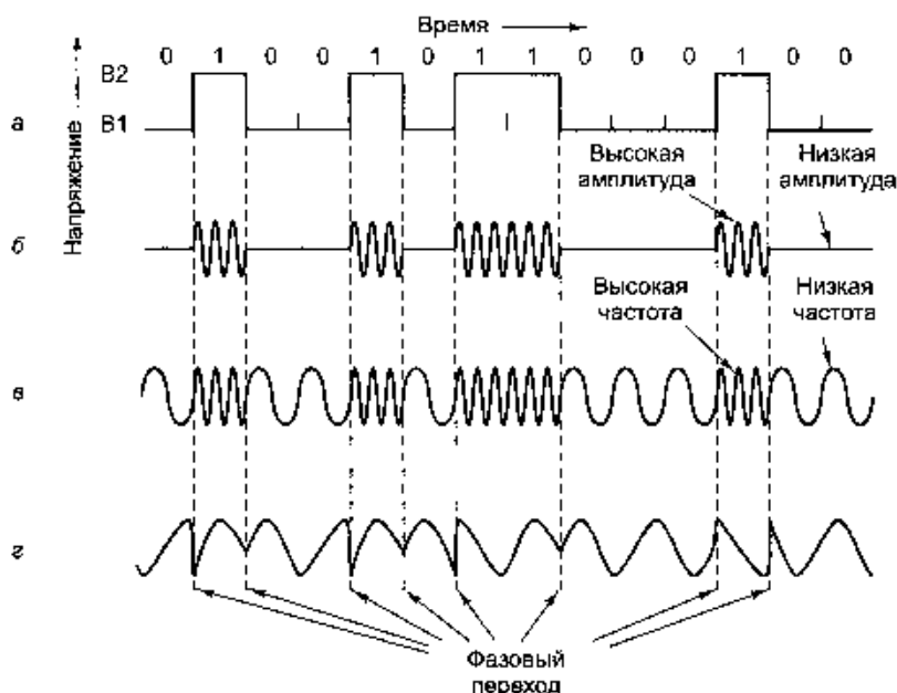
Рис. 2.33. Последовательная передача двоичного числа 01001011000100 по телефонной линии: двухуровневый сигнал (а); амплитудная модуляция (б); частотная модуляция (в); фазовая модуляция (г)
