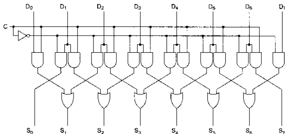
Рис. 3.15. Схема сдвига
