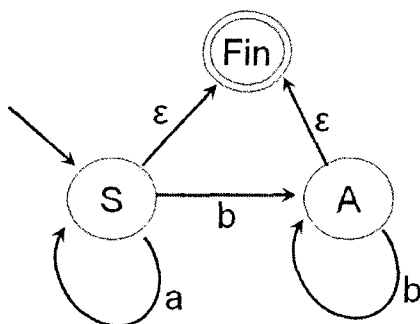
Рис. 5.3. Автомат, построенный для данной праволинейной грамматики
