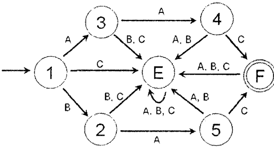
Рис. 2.7. Автомат с полным набором правил
