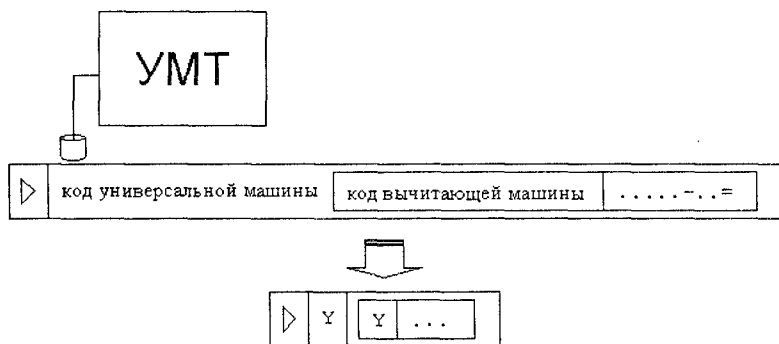
Рис. 10.18. Эмуляция универсальной машины универсальной машиной Тьюринга
