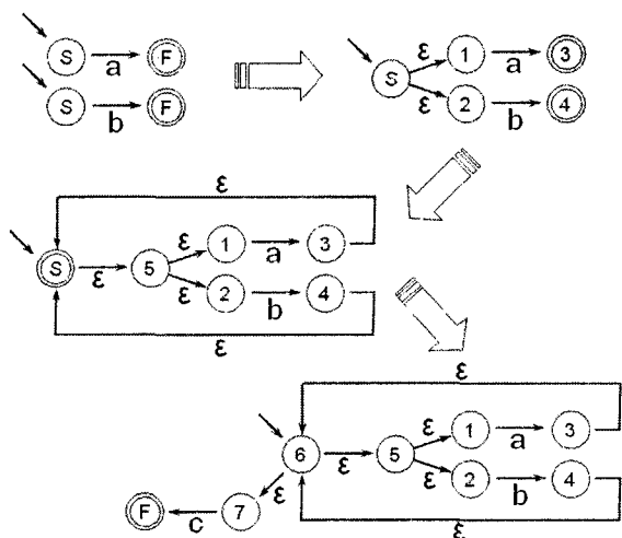
Рис. 3.5. Конструирование автомата для выражения (a \cup b)^*c
