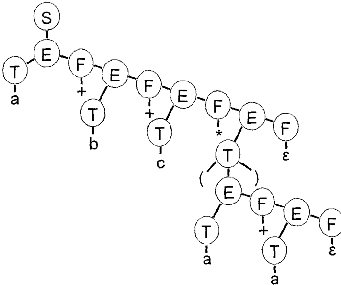
Рис. 7.6. Дерево разбора строки a+b+c*(a+b) , случай LL(1) грамматики
