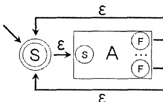
Рис. 3.4. Автомат, соответствующий замыканию Клини
