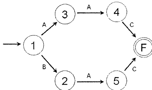
Рис. 2.5. Эквивалентность состояний
