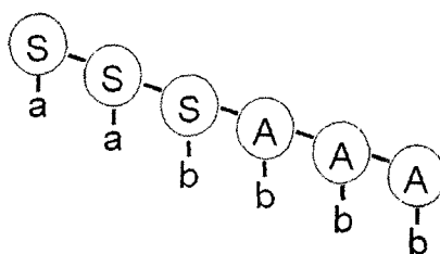
Рис. 7.4. Дерево разбора строки aabbabb
