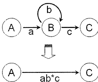
Рис. 3.6. Замена состояния регулярным выражением
