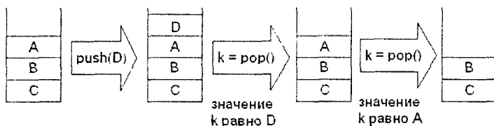
Рис. 6.1. Принцип работы стека
