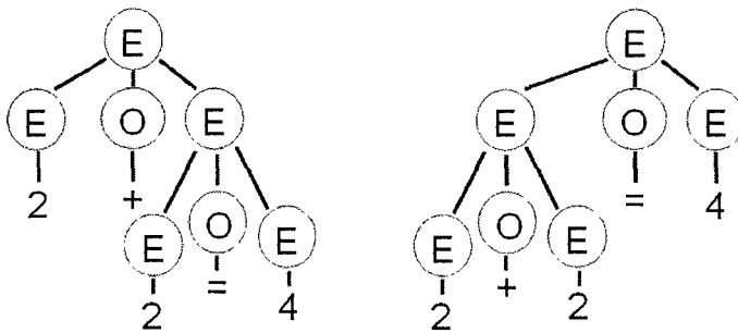
Рис. 7.3. Деревья разбора строки 2+2=4
