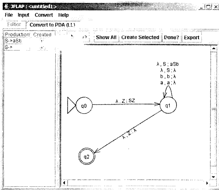
Рис. 6.5. Конструирование магазинного автомата по заданной грамматике (JFLAP)
