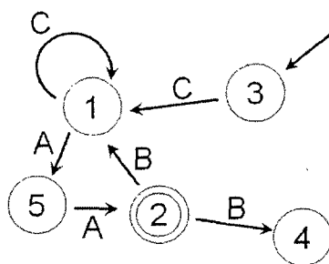
Рис. 2.2. Представление конечного автомата с помощью графа
