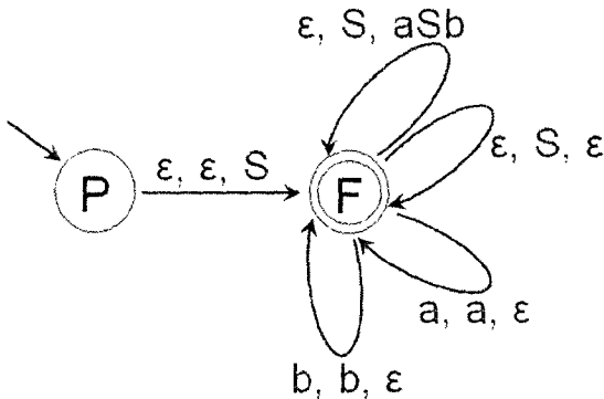
Рис. 6.4. Готовый автомат
