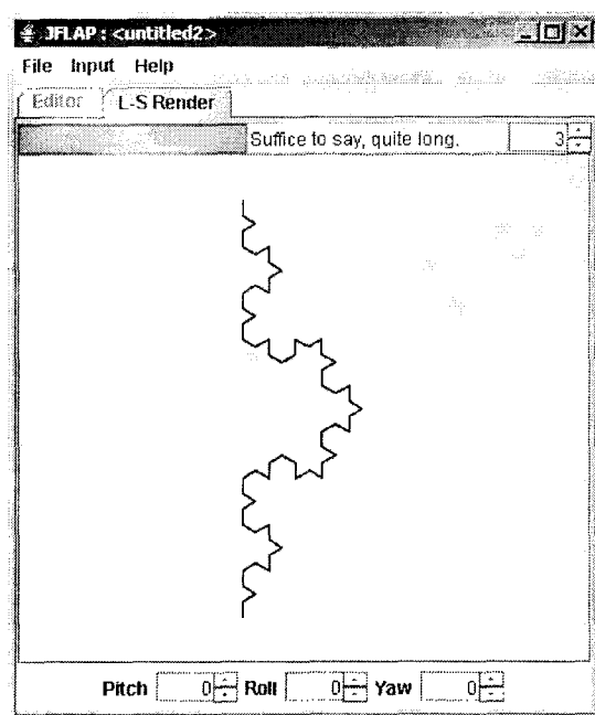
Рис. 9.8. Кривая Коха третьего порядка
