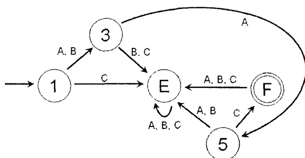
Рис. 2.8. Минимизированный автомат
