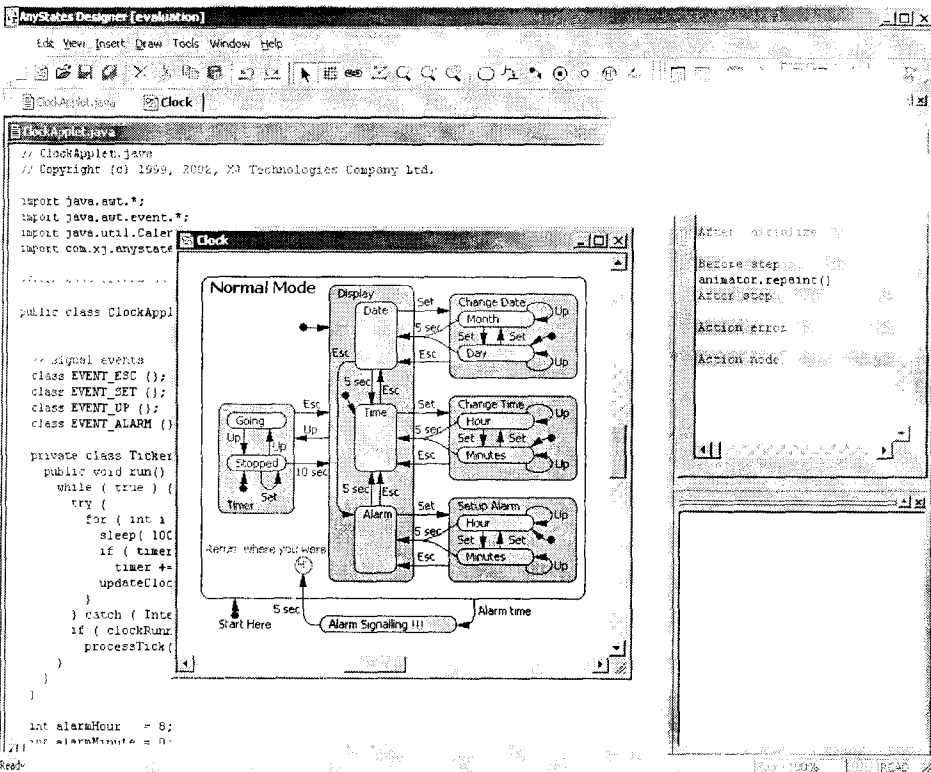
Рис. 4.3. Окно редактора AnyStates
