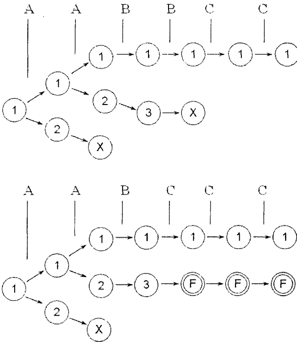
Рис. 2.10. Обработка строк AABVCC и AABCCC автоматом
